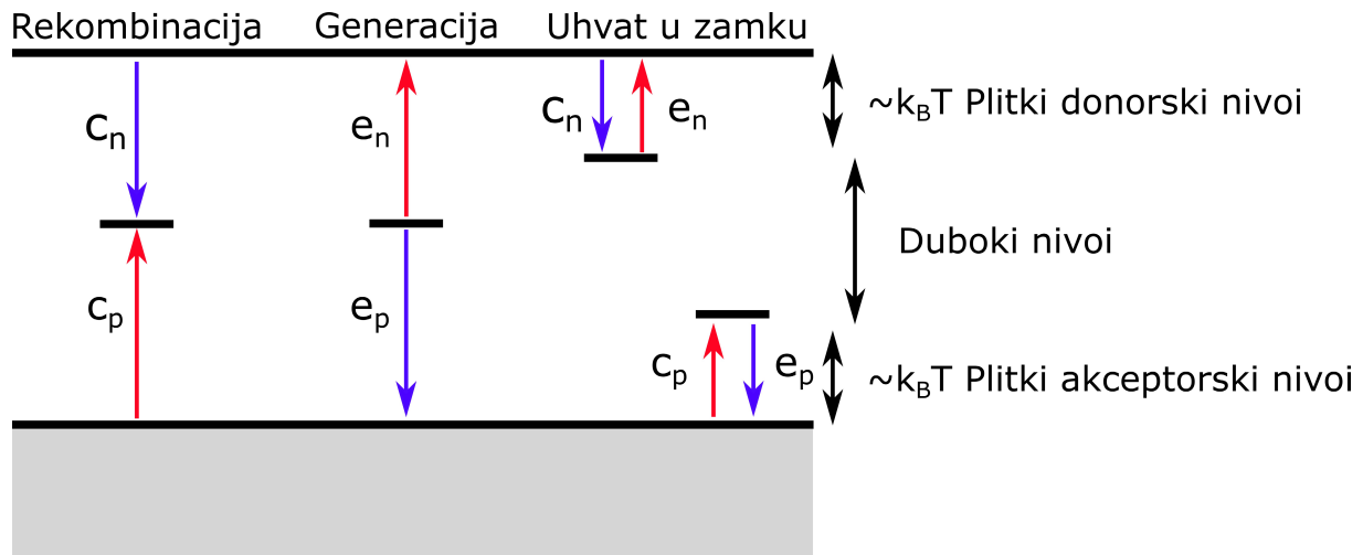
Slika 5. Shematski prikaz interakcije dubokih nivoa s vodljivom i valentnom vrpcom. Vjerojatnosti emisije i uhvata elektrona (šupljina) su redom označene s e_n i c_n ( e_p i c_p ).
