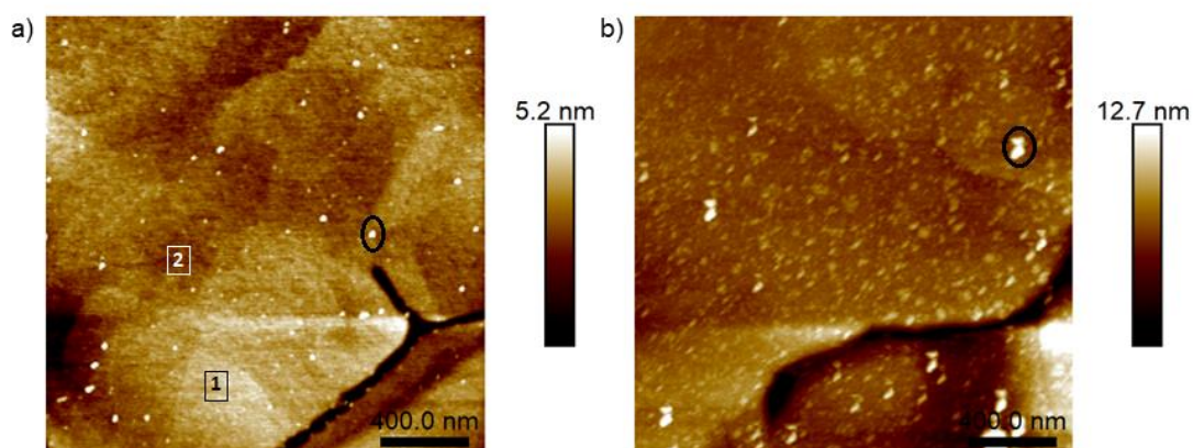
Slika 24. 2 \mu\text{m} \times 2 \mu\text{m} AFM slike molekularnih slojeva nastalih uranjanjem supstrata zlata (111) na 24 sata u otopinu spoja 2c koncentracije a) 1 \times 10^{-3} mol \text{dm}^{-3} i b) 1 \times 10^{-6} mol \text{dm}^{-6} .
