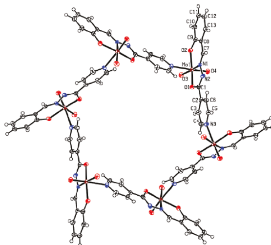
Slika 13. Struktura heksamernog kompleksa [\text{MoO}_2(\text{SIH})]_6 11
