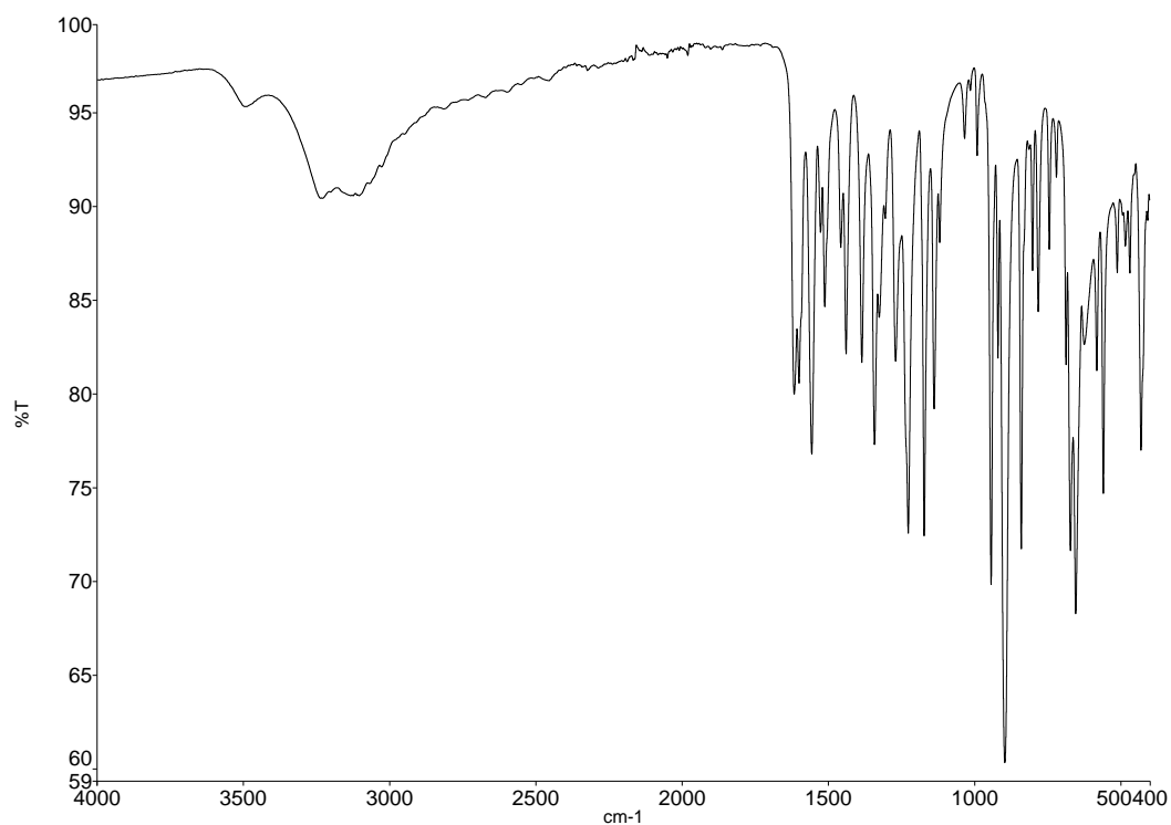
Slika D13. Infracrveni spektar kompleksa [\text{MoO}_2(4\text{OHSal}-4\text{HBOH})(\text{H}_2\text{O})]
