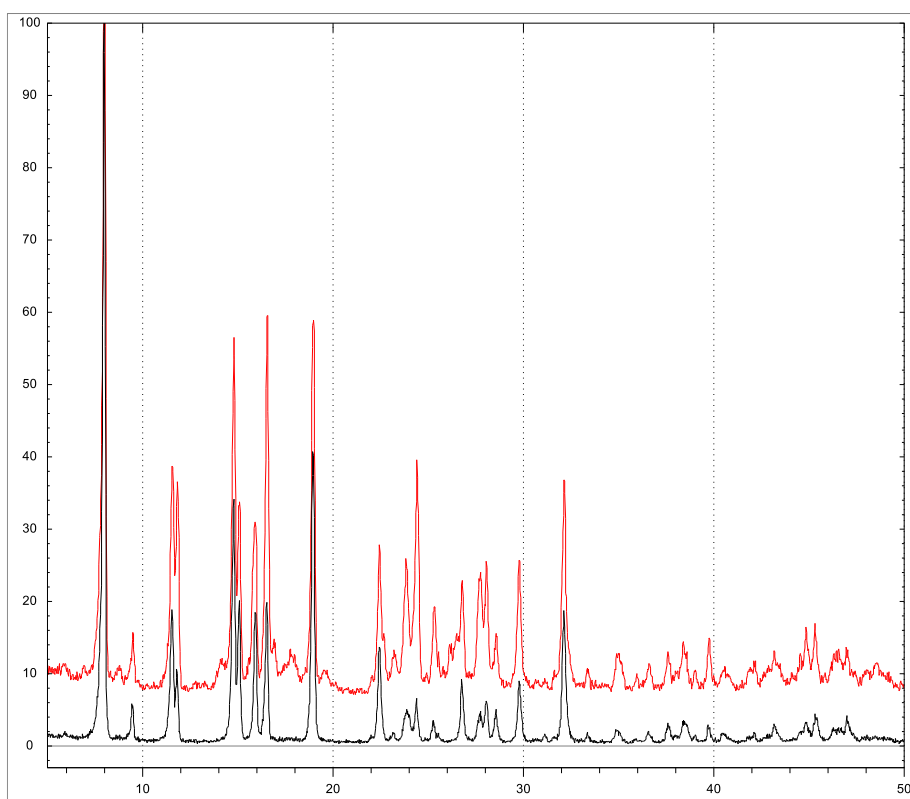
Slika 19. Usporedba difraktograma prahova polimernog spoja [\text{MoO}_2(4\text{OHSal}-4\text{HBOH})]_n dobivenog sintezom uz reflux (crno) i solvotermalnom isntezom (crveno)
