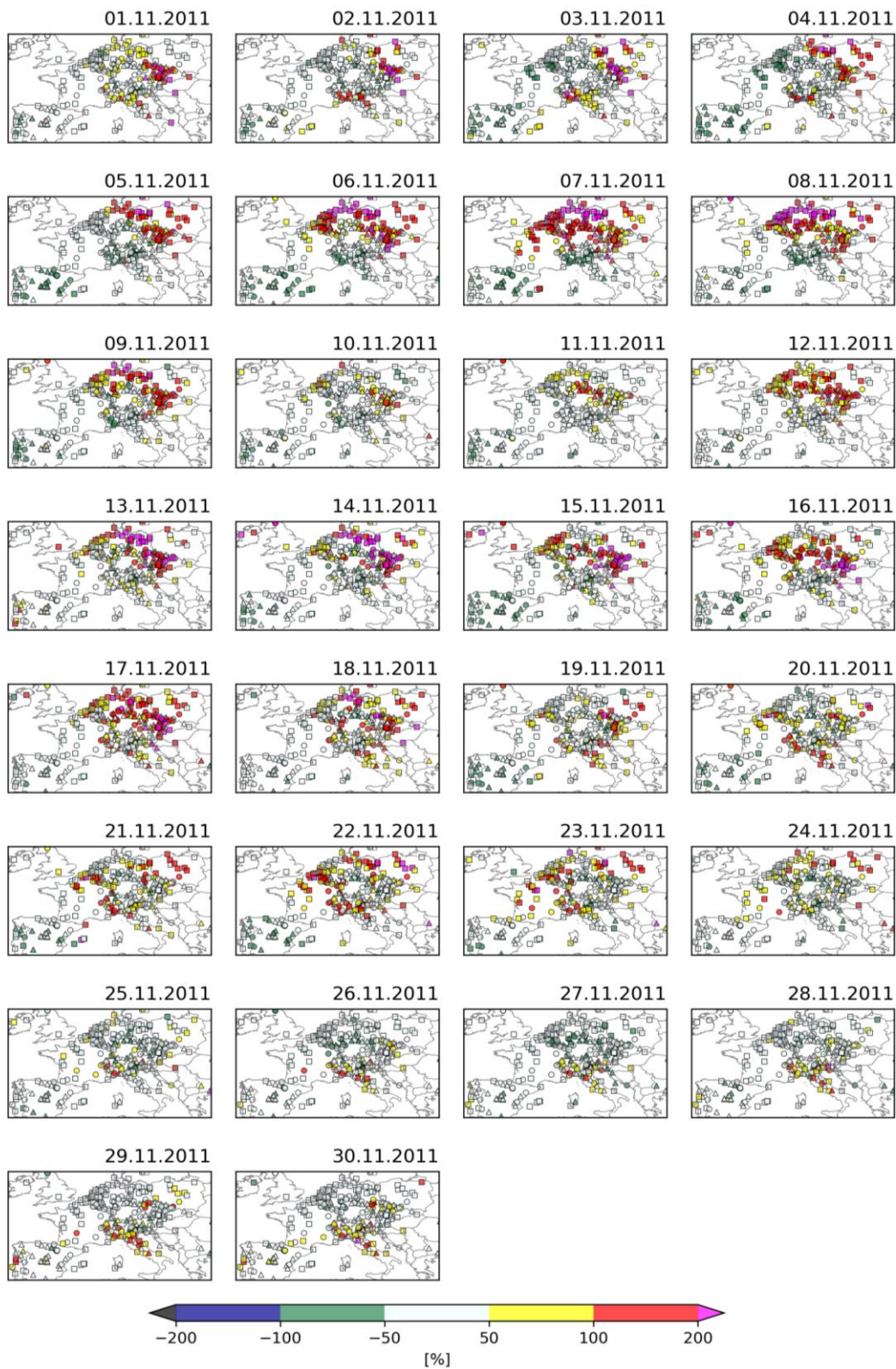
Slika D1. Prostorni prikaz razlika ( DF ) između (PM_{10})_d i (PM_{10})_a koncentracija (relacija 10) iznad Europe tijekom studenoga 2011. godine.
