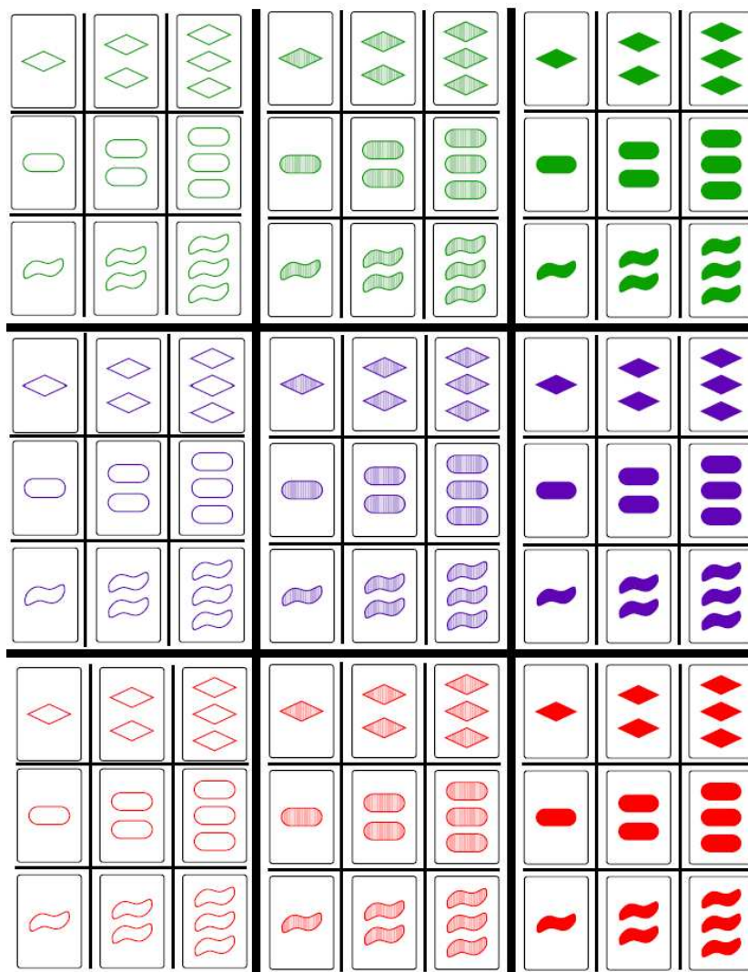
Slika 1.12: SET
