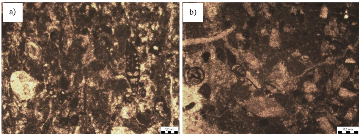
Sl. 10. a) Biplanatna peneropliformis Hamaoui i rothalidne foraminifere; b) Pseudolituonella reicheli Marie (uzorak P1-05)
