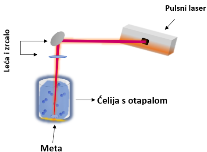
Slika 2.14: Postav za lasersku ablaciju
