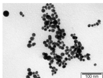
Slika 3.40: TEM snimka zlatnih nanočestica Povećanje x300 000
