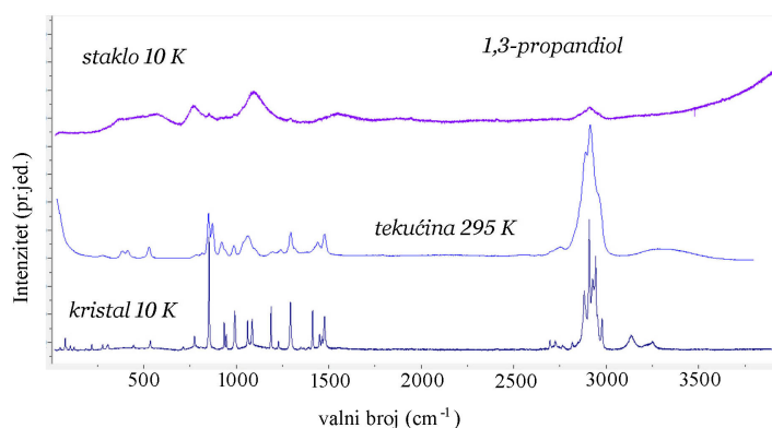
Slika 3.36: Ramanovi spektri za različita agregatna stanja 1,3 propandiola. Iz arhive Lab. za molekulska fiziku i sinteze novih materijala, IRB
