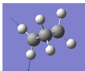
(a) Amplitude atoma u vibraciji istezanja
