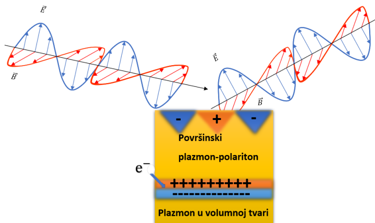
Slika 1.4: Pobuđivanje plazmona u volumnoj tvari uzrokuju slobodni elektroni, dok PSPP pobuđuje vanjski propagirajući elektromagnetski val.
