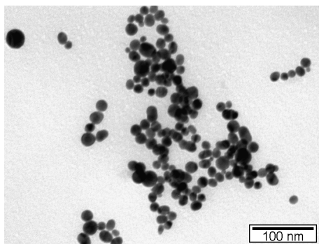
Slika 2.24: TEM slika uzorka koloida zlata
