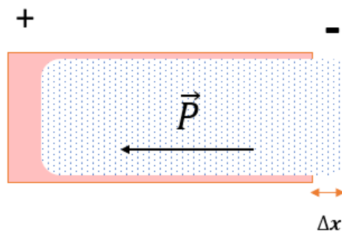
Slika 1.3: Titranje plazme
