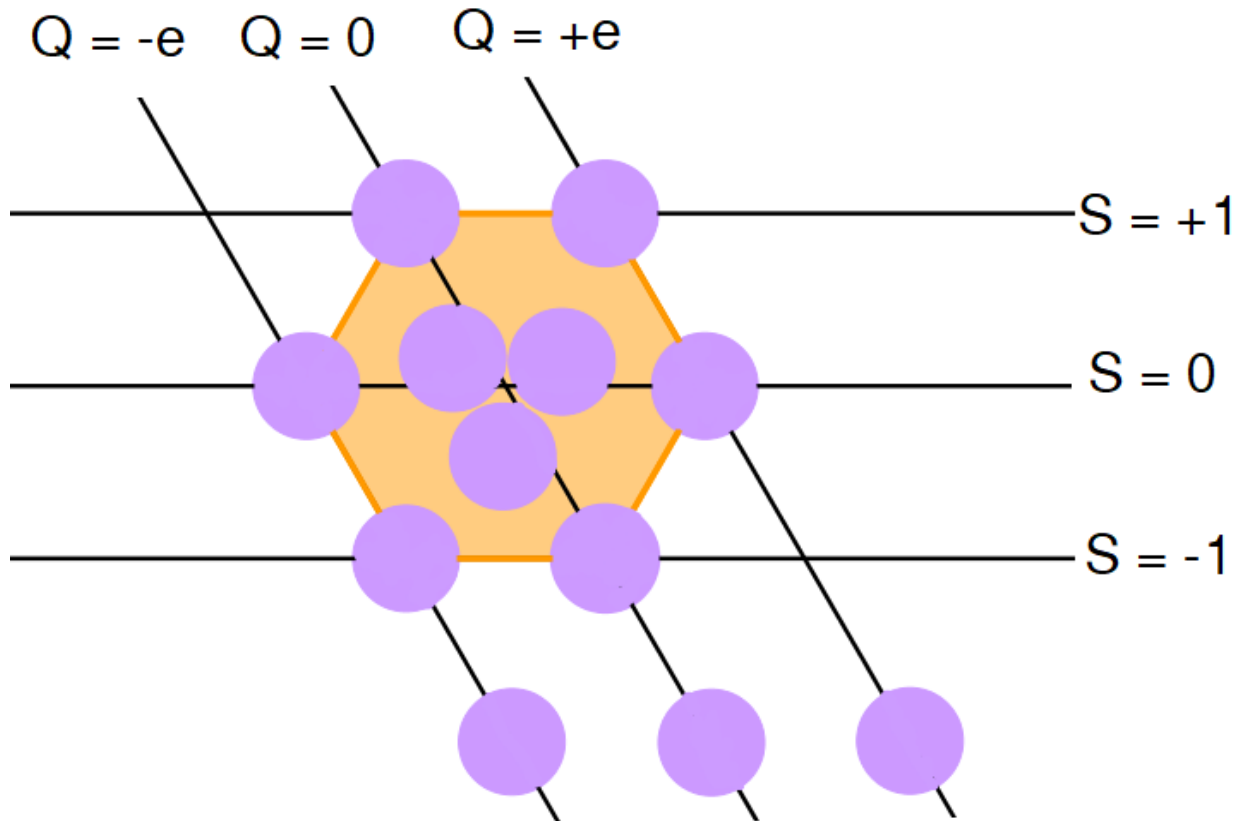
Slika 72 – „Mezonski šesterokut“
