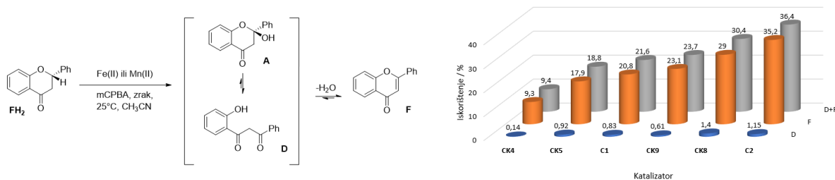
Slika 63. Usporedba aktivnosti različitih kompleksa željeza(II) i mangana(II). Uvjeti: [M^{II}] = 5 \text{ mmol dm}^{-3} , [FH_2] = 100 \text{ mmol dm}^{-3} i [mCPBA] = 500 \text{ mmol dm}^{-3} u CH_3CN pri 25^\circ C .
