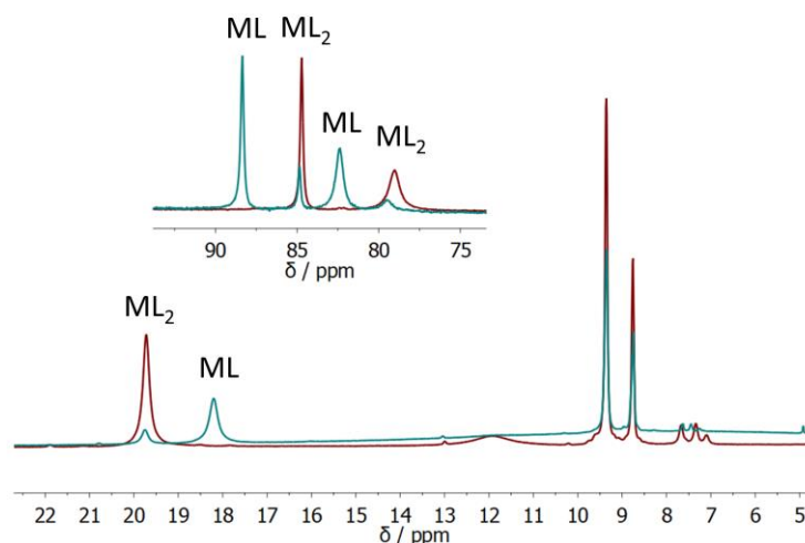
Slika 38. Paramagnetski 1 H NMR (CD 3 CN) liganda AL1 i Co(BF 4 ) 2 u omjerima 2:1 (crveno) i 1:4 (plavo).
