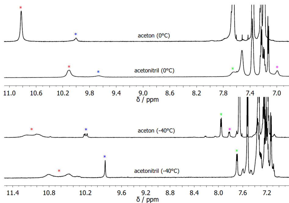
Slika 79. 1 H NMR spektri (aromatski dio) kompleksa [Zn(Di 3 B) 2 ] 2+ . Pikovi amidnih skupina koje pripadaju imda skupini označeni su crveno i plavo, a pikovi amidnih skupina iz pokrajnjeg lanca označeni su zeleno i ljubičasto.
