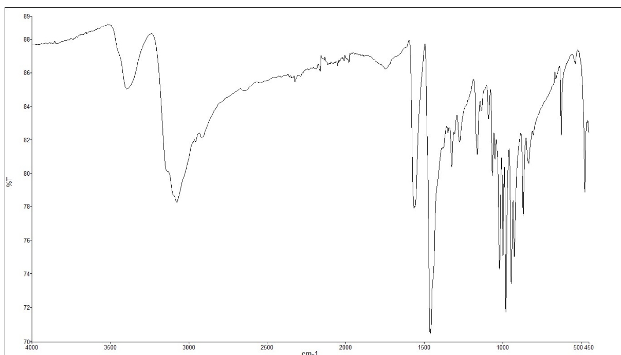
Slika D10. IR spektar H_2(DPOH)[CuBr_4] . Spoj je dobiven otopinskom sintezom uz acetonitril kao otapalo
