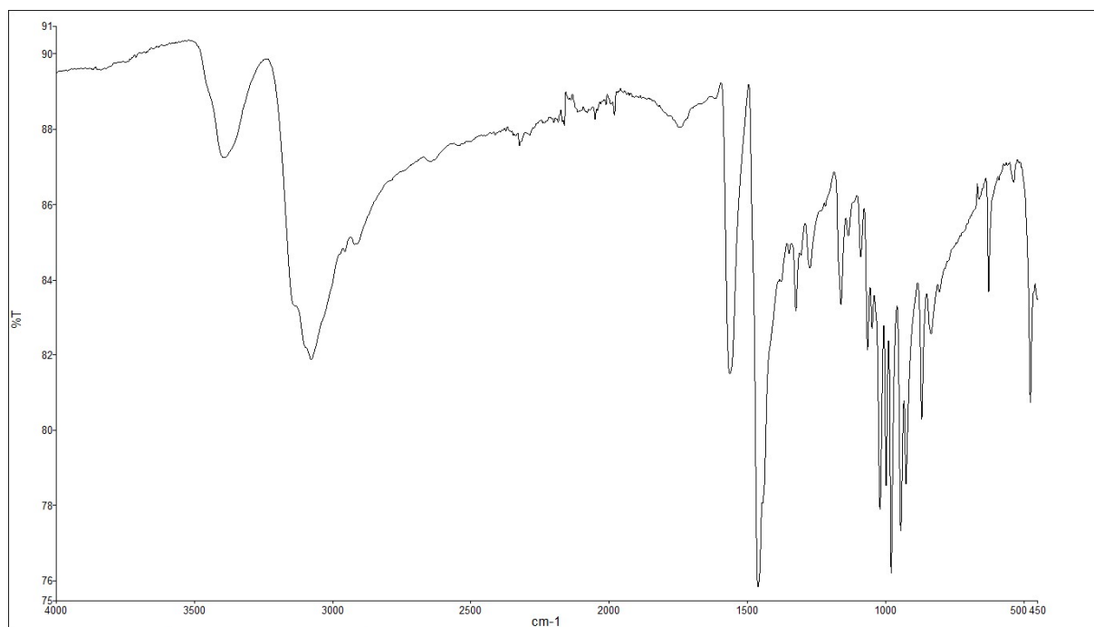
Slika D9. IR spektar H_2(DPOH)[CuBr_4] . Spoj je dobiven otopinskom sintezom uz etanol kao otapalo
