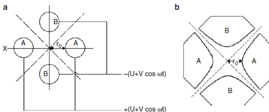
Slika 4. Poprečni presjek a) cilindrično oblikovanih elektroda i b) hiperbolično oblikovanih elektroda kvadrupola. 4
