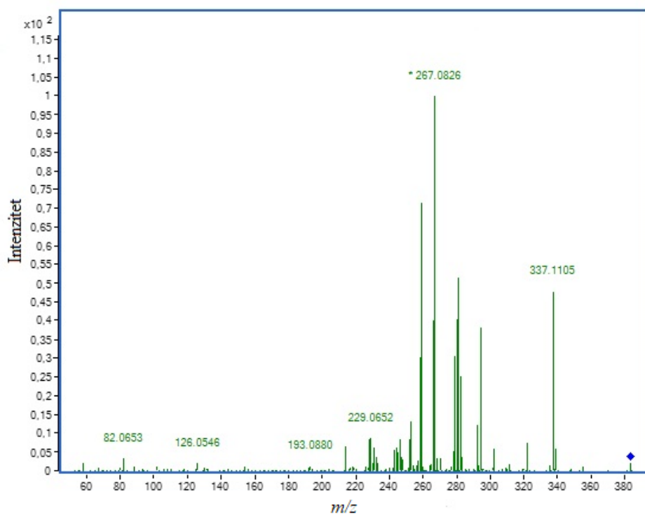
Slika D6. MS/MS spektar masa iona [LOR+H]^+ pri kolizijskom potencijalu od 40 V. Ionizacijska tehnika ESI+.
