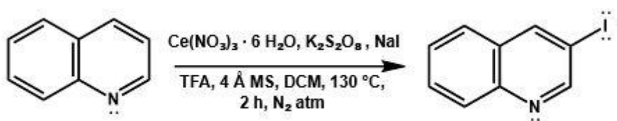
Slika 13. Shema uvođenja halogena na piridinski prsten kinolina
