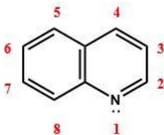
Slika 1. Strukturna formula i numeriranje atoma molekule kinolina
