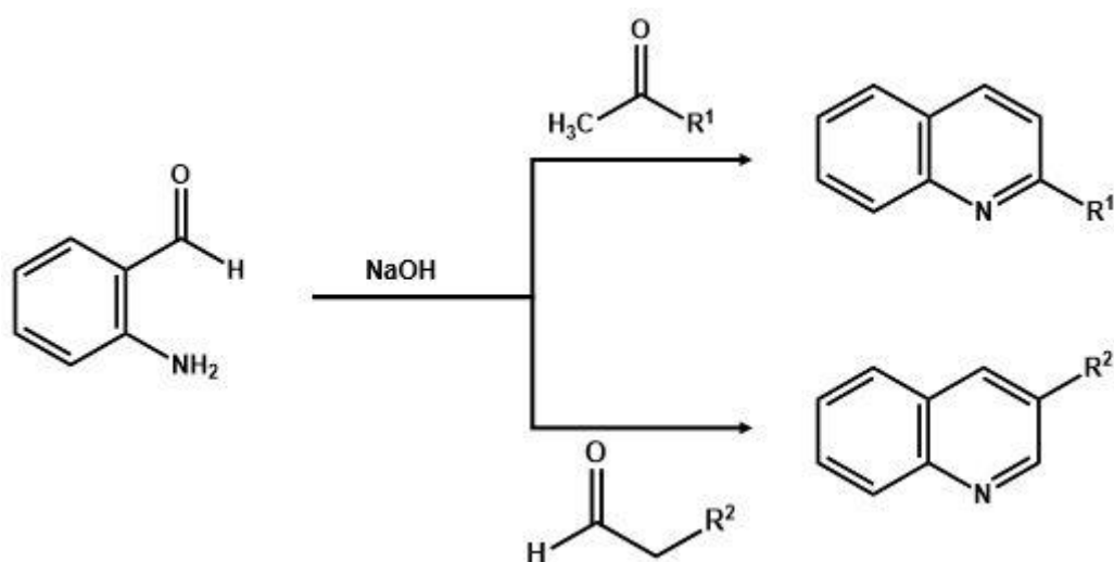
Slika 18. Shema reakcije kondenzacije 2-aminobenzaldehida s različitim metil-ke-tonima i aldehydima
