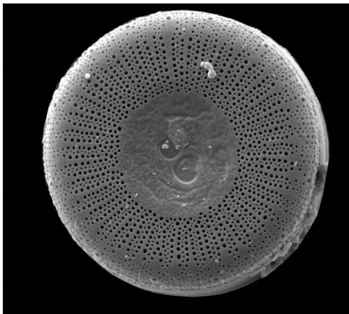
Slika 4. Cyclotella plutvicensis , dijatomeja reda Centrales
