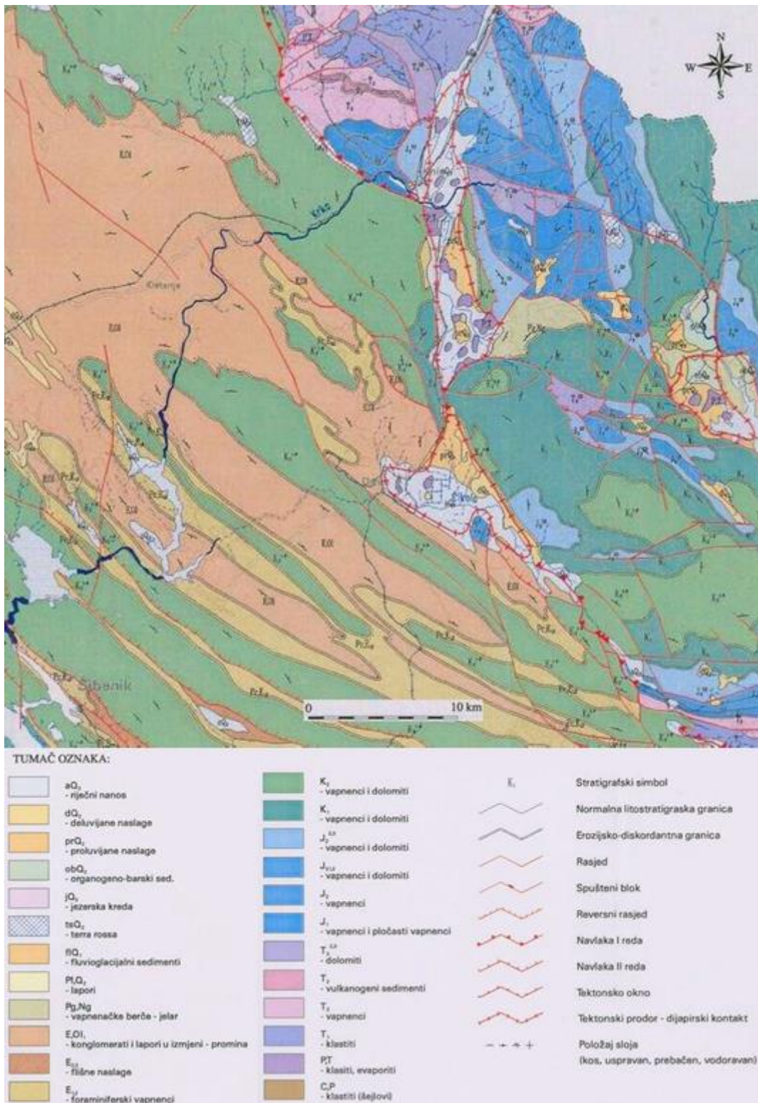
Slika 3. Geološka karta šireg porječja Krke (preuzeto iz Kapelj 2002).
