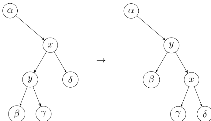
Slika 2.1: Desna rotacija
