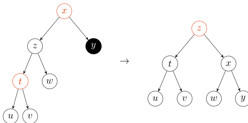
Slika 2.6: 2. slučaj
