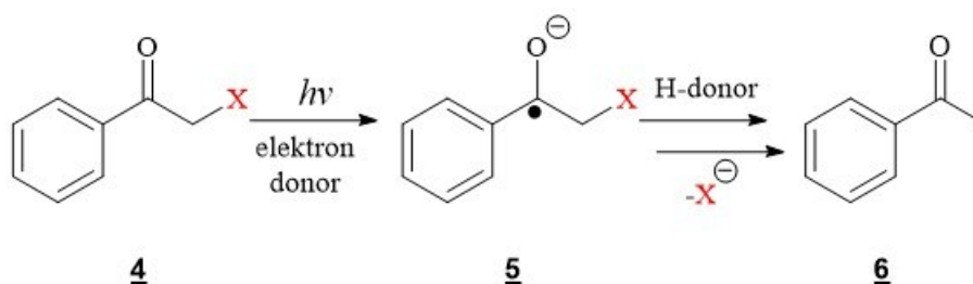
Shema 3. Primjer fotokemijske reakcije aromatskog ketona u prisutnosti donora elektrona te otpuštanje izlazne skupine X. 2
