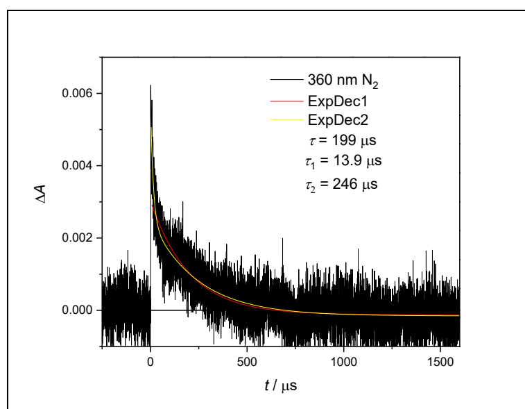
Slika D30. Opadanje intenziteta tranzijentne apsorpcije na 360 nm za spoj 7 u N_2 -propuhanoj otopini CH_3CN .
