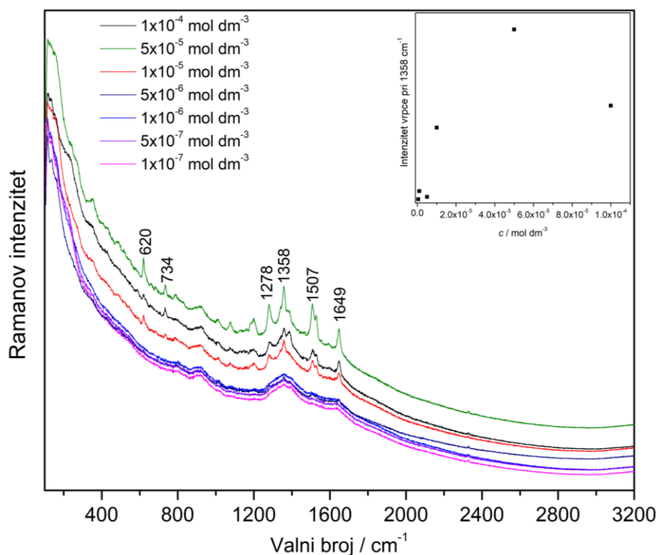
Slika 16. SERS spektri spoja RB različitih koncentracija u svježe pripremljenom koloidu srebra, AgNP_svježi, pri valnoj duljini pobude 785 nm, snaga lasera 300 mW
