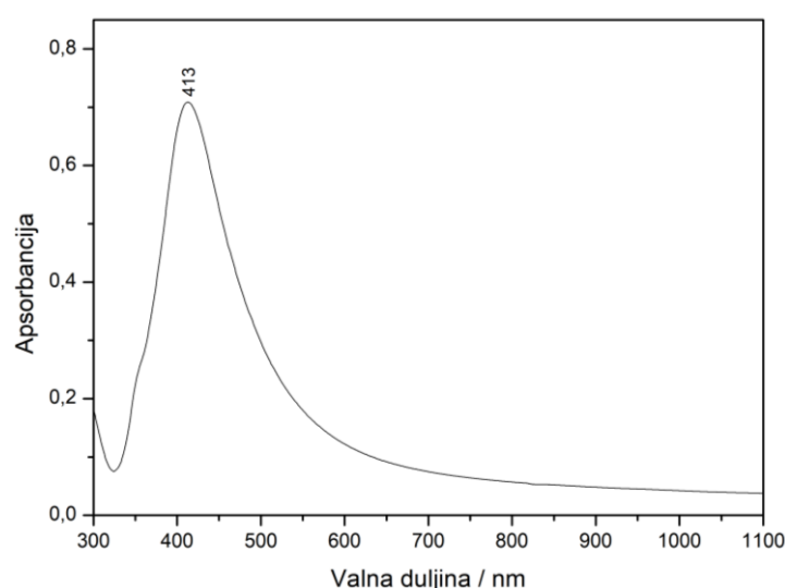
Slika 7. UV/Vis spektr AgNP svježeg koloida
