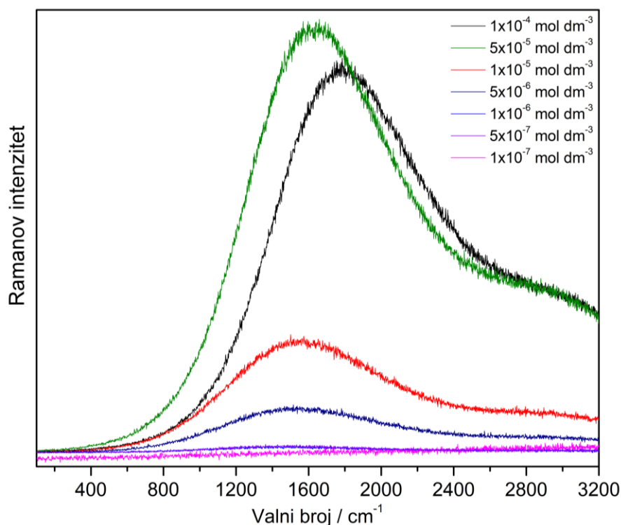
Slika 15. SERS spektri spoja RB različitih koncentracija u svježe pripremljenom koloidu srebra, AgNP_sveježi, pri valnoj duljini pobude 532 nm, snaga lasera 0,1 \mu W
