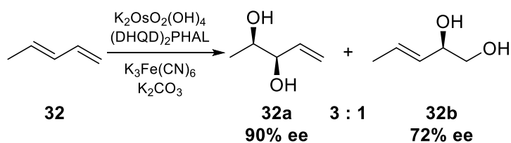
Shema 24. Sharplessova dihidroksilacija konjugiranog olefina 32
