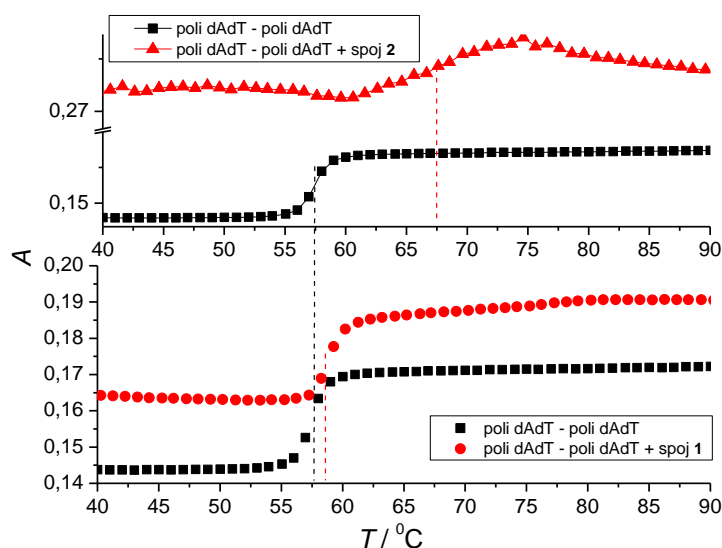
Slika 23. Krivulje temperature mekšanja polinukleotida poli dAdT – poli dAdT ( c(\text{poli dAdT} - \text{poli dAdT}) = 2,5 \times 10^{-5} \text{ mol L}^{-1} , r_{[\text{spoj}]/[\text{polinukleotid}]} = 0,3 ) snimljene u puferu natrijeva kakodilata (pH 7,0; I = 0,05 \text{ mol L}^{-1} ) nakon dodatka spojeva 1 i 2 . Greška u vrijednostima \Delta T_m iznosi \pm 0,5 \text{ }^\circ\text{C} . Prve derivacije sigmoidnih krivulja ovisnosti apsorbancije o temperaturi prikazane su u Dodatku.
