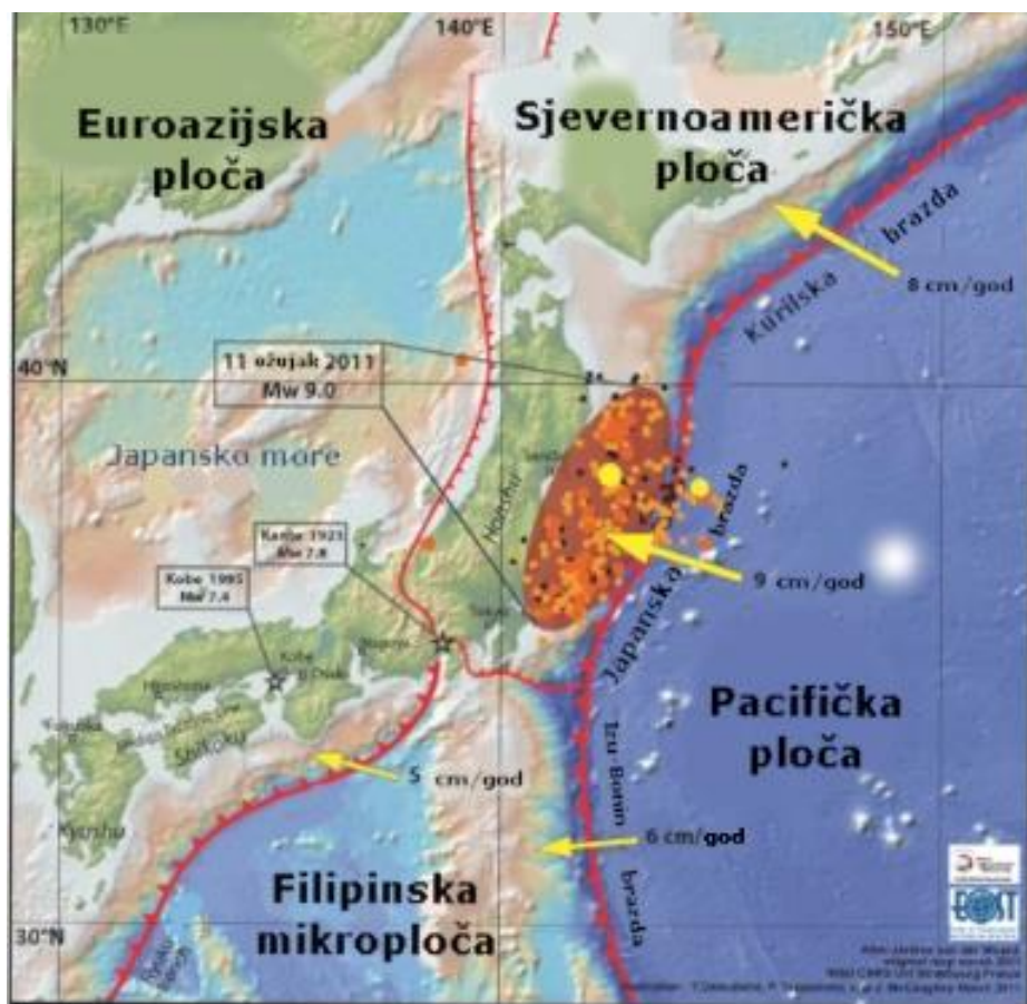
Sl.6. Položaj i smjer kretanja litosfernih ploča na području Japana te epicentar velikog potresa i najvećeg naknadnog potresa
