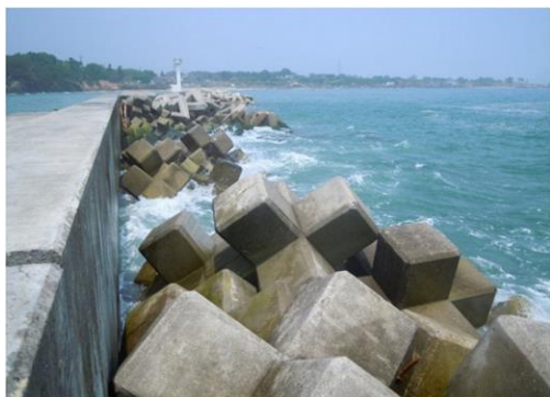
Sl.12. Sustav za zaštitu od tsunamija Izvor: Esteban i dr. (2014)
