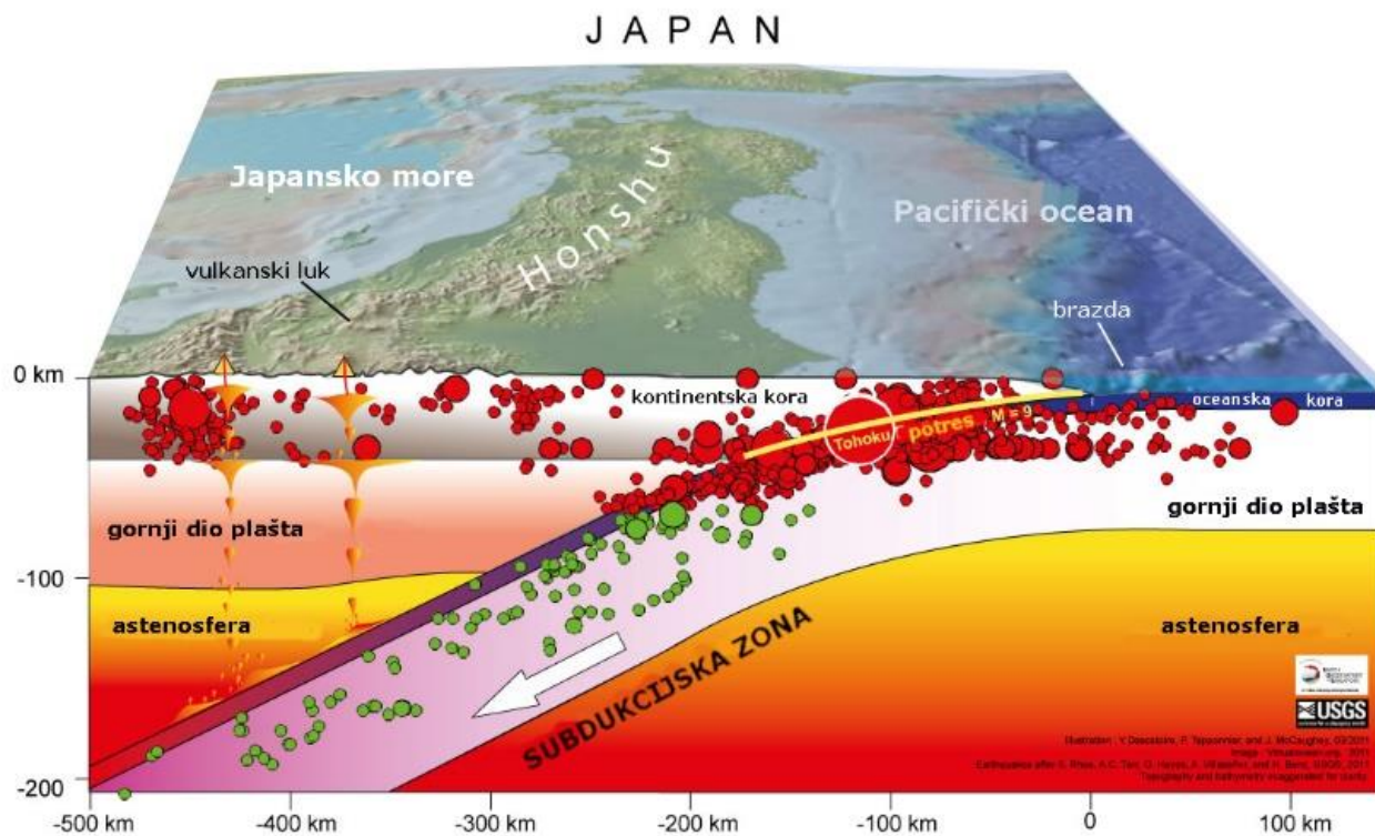
Sl.1. Subdukcija Tihooceanske ploče pod Euroazijsku na području otoka Honshu
