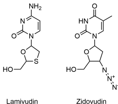
Slika 15. Strukture lamivudina i zidovudina.
