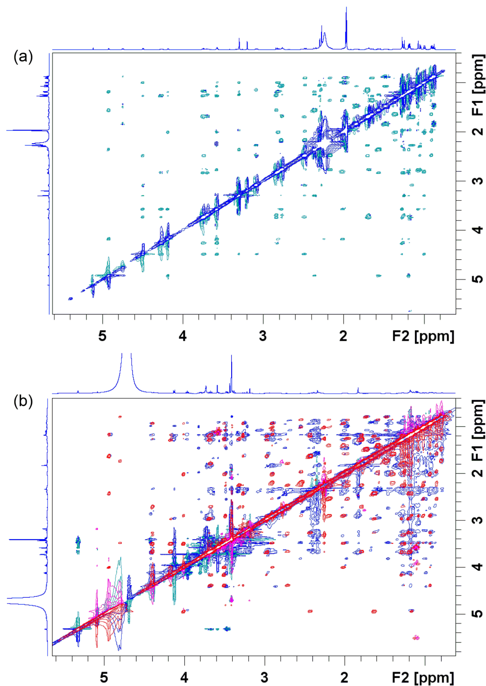
Slika 11. a) Spektar NOESY 4''-aminopropil-azitromicina u acetonitrilu- \text{d}_3 prije dodatka ribosoma iz E. coli ; b) spektar NOESY (ružičasti i crveni signali) i trNOESY (plavi i zeleni signali) istog spoja u puferu \text{tris-d}_{11} prije odnosno nakon dodatka ribosoma iz E. coli . 4
