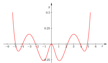
Slika 2.47: Greška interpolacijskog polinoma stupnja 6
