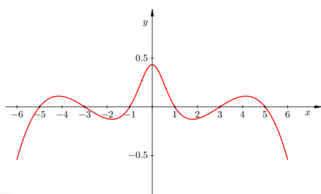
Slika 2.24: Greška interpolacijskog polinoma stupnja 5
