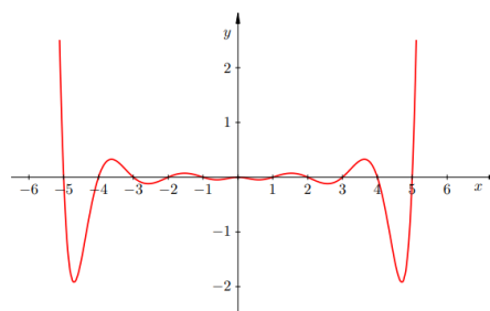
Slika 2.27: Greška interpolacijskog polinoma stupnja 10
