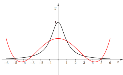
Slika 2.13: Interpolacijski polinom stupnja 5
