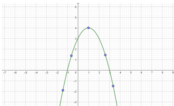
Slika 0.2: Primjer interpolacije kvadratnom funkcijom
