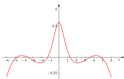
Slika 2.46: Greška interpolacijskog polinoma stupnja 5
