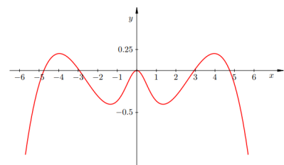
Slika 2.45: Greška interpolacijskog polinoma stupnja 4
