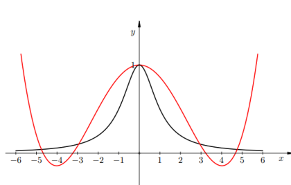
Slika 2.34: Interpolacijski polinom stupnja 4
