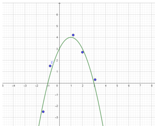
Slika 0.1: Primjer aproksimacije kvadratnom funkcijom
