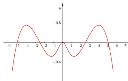
Slika 2.23: Greška interpolacijskog polinoma stupnja 4
