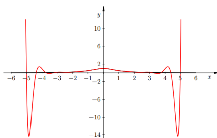
Slika 2.19: Interpolacijski polinom stupnja 16
