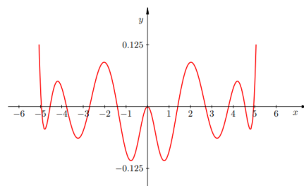
Slika 2.49: Greška interpolacijskog polinoma stupnja 10
