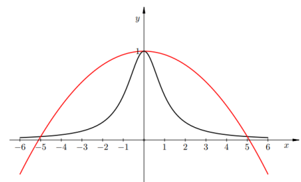
Slika 2.10: Interpolacijski polinom stupnja 2
