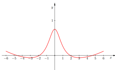
Slika 2.44: Greška interpolacijskog polinoma stupnja 3
