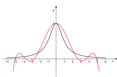
Slika 2.36: Interpolacijski polinom stupnja 6
