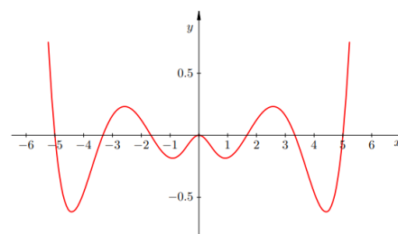
Slika 2.25: Greška interpolacijskog polinoma stupnja 6
