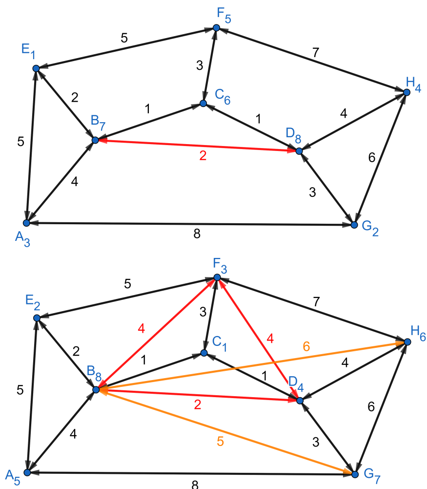
Slika 4.3: Primjer utjecaja redoslijeda kontrakcija vrhova na broj dodanih bridova prečaca. Crnom bojom označeni su početni bridovi, dok su bridom u boji označeni dodani prečaci.
