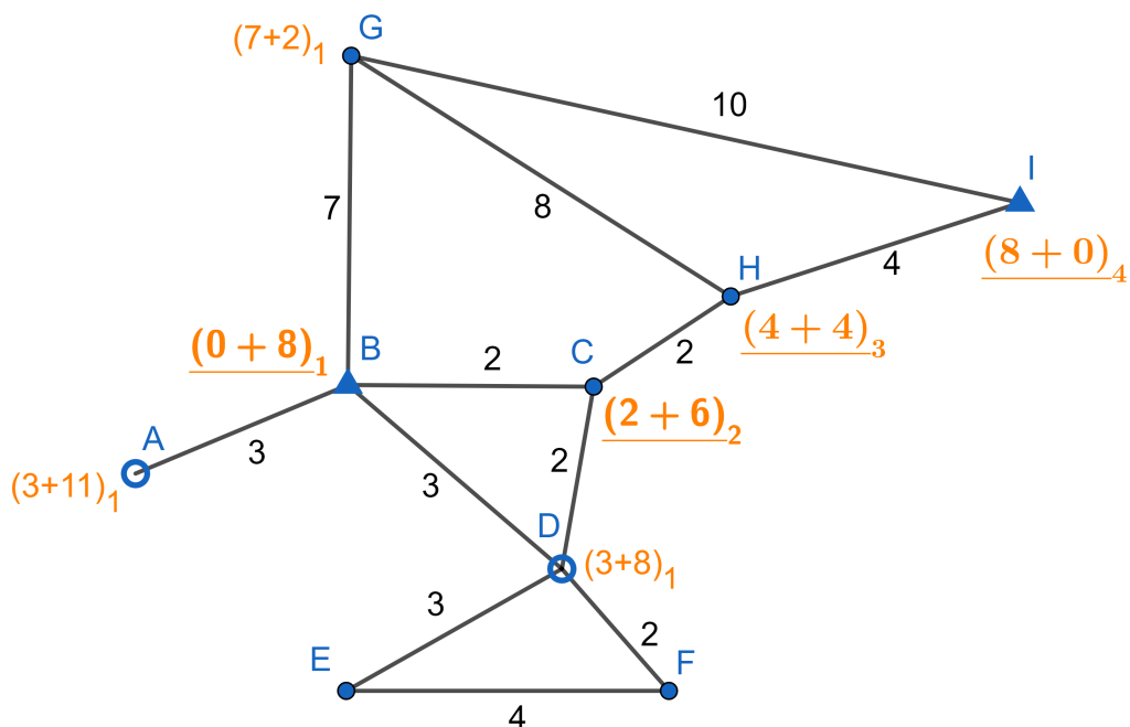
Slika 5.2: Primjer faze upita ALT algoritma. Vrhovi orientiri su A i D te se traži d_G(B, I) .
