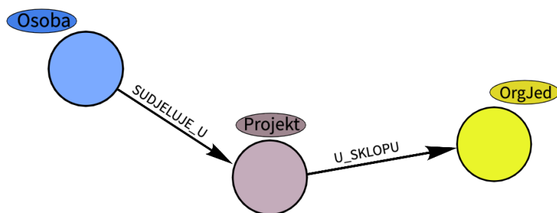
Slika 4.2: Model grafa
