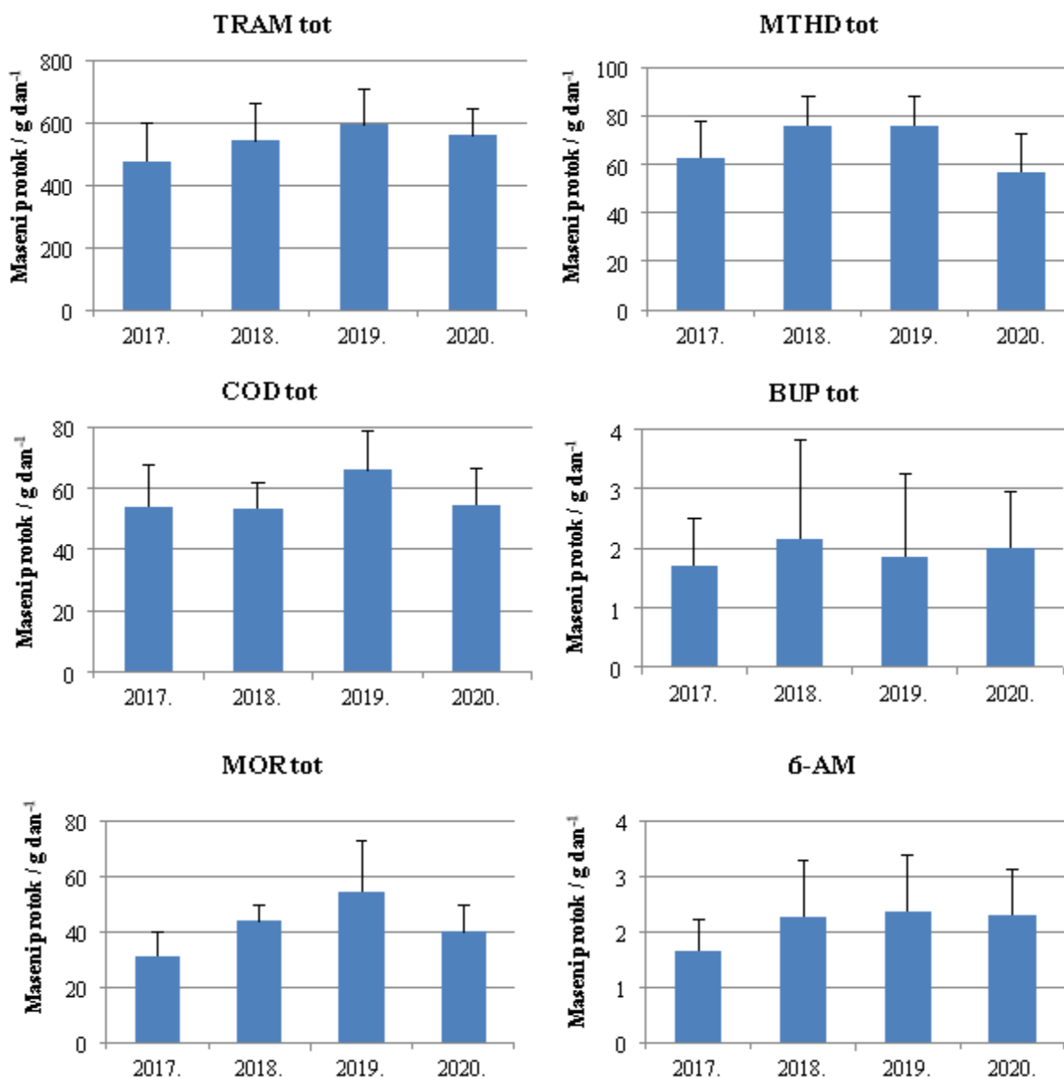
Slika 22. Višegodišnje promjene srednjih vrijednosti dnevnih masenih protoka odabranih biomarkera opioidnih analgetika u četverogodišnjem razdoblju (od 2017. do 2020.); ukupni tramadol ( \text{TRAM}_{\text{tot}} ), metadon ( \text{MTHD}_{\text{tot}} ), buprenorfin ( \text{BUP}_{\text{tot}} ), kodein ( \text{COD}_{\text{tot}} ), morfin ( \text{MOR}_{\text{tot}} ) i 6-acetilmorfin (6-AM)
