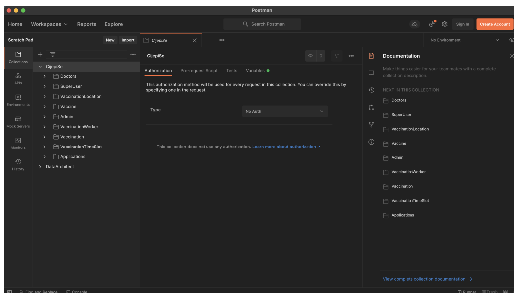
Slika 3.21: Postman sučelje
