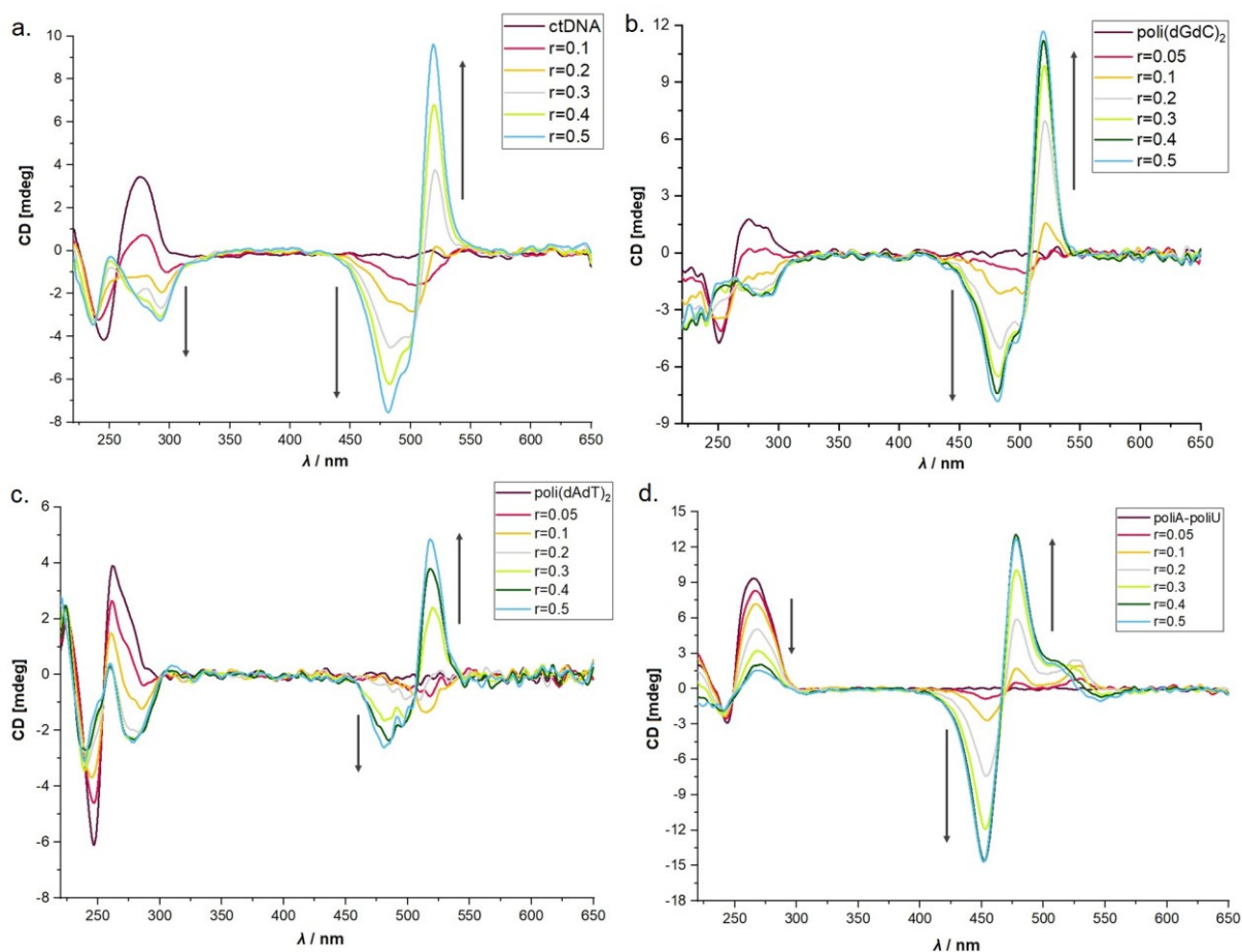
Slika 28. CD titracija a. ctDNA, b. poly(dGdC) 2 , c. poly(dAdT) 2 i d. poly A-poly U ( c = 3 \times 10^{-5} \text{ mol dm}^{-3} ) sa spojem AK-3 pri različitim molarnim omjerima r_{\text{[spoju] / [polinukleotid]}} u puferu natrijeva kadolidata ( I = 0,05 \text{ mol dm}^{-3} , pH 7,00)
