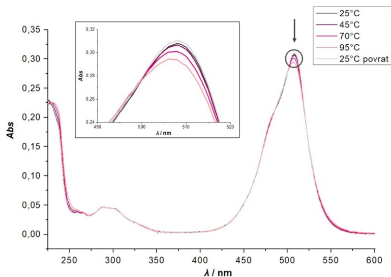
Slika 20. Temperaturna ovisnost UV/Vis spektra spoja AK-1 ( c = 4 \times 10^{-6} \text{ mol dm}^{-3} ) u puferu natrijeva kakovilata ( I = 0,05 \text{ mol dm}^{-3} , \text{pH} = 7,00 )
