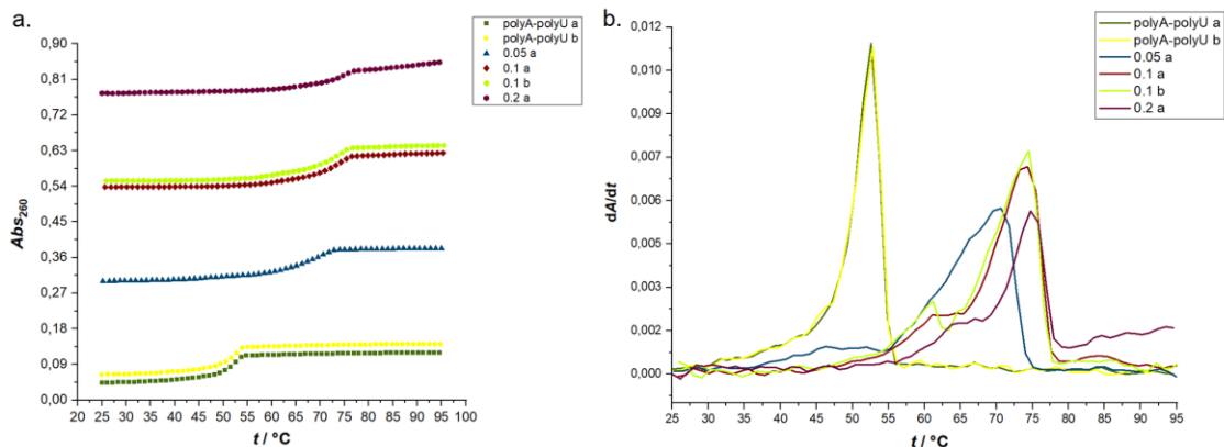
Slika D23. a. krivulja mekšanja poli A-poli U ( c = 1,26 \times 10^{-2} \text{ mol dm}^{-3} ) uz dodatak AK-2 u omjerima r_{[spoj]}/[polinukleotid] = 0,05, 0,1 \text{ i } 0,2 u puferu natrijeva kakodilata ( I = 0,05 \text{ mol dm}^{-3} , pH 7,00) b. prva derivacija derivacija denaturacijske krivulje poli A-poli U
