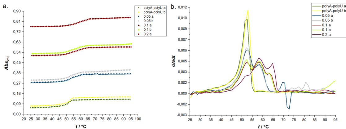
Slika D24. a. krivulja mekšanja poli A-poli U ( c = 1,26 \times 10^{-2} \text{ mol dm}^{-3} ) uz dodatak AK-3 u omjerima r_{[spoj]}/[polinukleotid] = 0,05, 0,1 \text{ i } 0,2 u puferu natrijeva kakodilata ( I = 0,05 \text{ mol dm}^{-3} , pH 7,00) b. prva derivacija derivacija denaturacijske krivulje poli A-poli U
