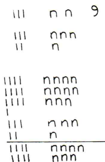
Slika 3.5: Oduzimanje 123 - 45 = 78 u Egiptu (preuzeto iz [3], str. 12.)
