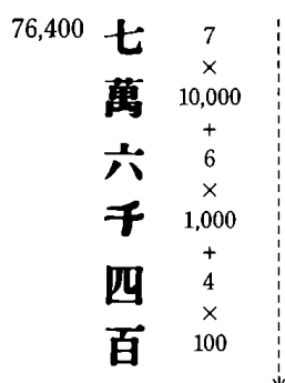
Slika 7.7: Tradicionalni zapis broja 76 400 (preuzeto iz [13], str. 281.)
