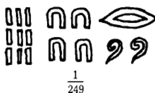
Slika 3.7: Zapisivanje egipatskog razlomka s velikim nazivnikom (v.[13], str. 169.)
