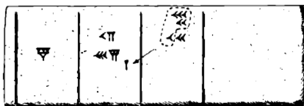
Slika 4.10: Prenosnje brojeva iz jednog stupca u drugi (preuzeto iz [13], str. 156.)
