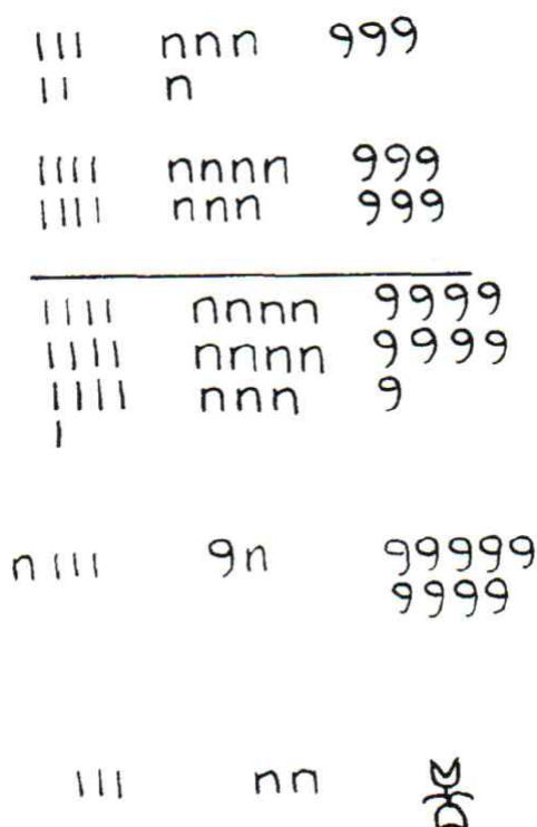
Slika 3.4: Zbrajanje 345 + 678 = 1023 u Egiptu (preuzeto iz [3], str. 12.)
