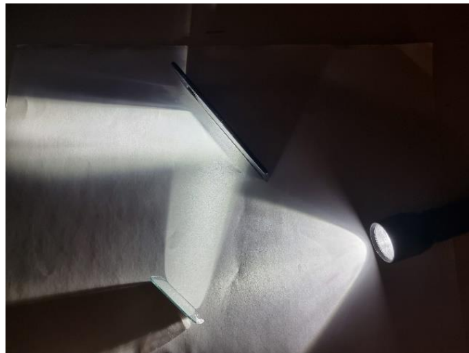
Slika 9. Refleksija svjetlosti
