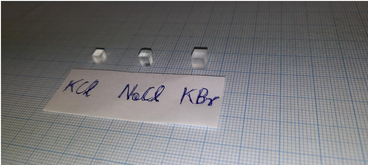
Slika 18. Kristali KCl , NaCl i KBr . Dimenzije kristala KCl su: x = 3.6 mm, y = 3.9 mm, z = 3.4 mm. Dimenzije kristala NaCl su: x = 4.0 mm, y = 3.9 mm, z = 4.8 mm. Dimenzije kristala KBr su: x = 4.8 mm, y = 5.3 mm, z = 4.9 mm ( x = duljina, y = širina, z = visina). Kristali su postavljeni između magneta tako da su duljine stranice kroz koje prolazi svjetlost za KCl = 3.6 mm, za NaCl = 4.0 mm, a za KBr = 4.8 mm.
