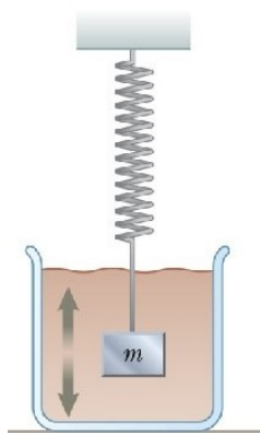
Slika 1.8: Sustav tijela na opruzi u fluidu [15]
