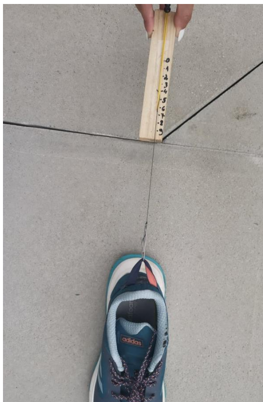
Slika 13. Mjerenje sile pri gibanju tenisice jednakom brzinom
