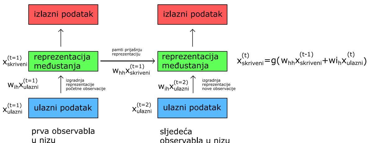
Slika 3.24: Shema principa rada ponavljajuće neuralne mreže
