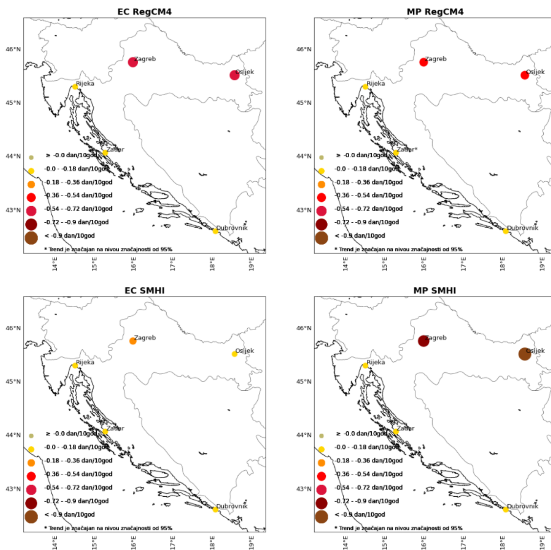
Slika 3.2.3: Karte Hrvatske s ucrtanim promatranim postajama i intervalima trenda izraženim u ^{\circ}\text{C}/10 god. za indeks ID za scenarij RCP 4.5 i različite kombinacije RCM-GCM. Postaja na kojoj je trend značajan na nivou značajnosti od 95 % označena je zvjezdicom.
