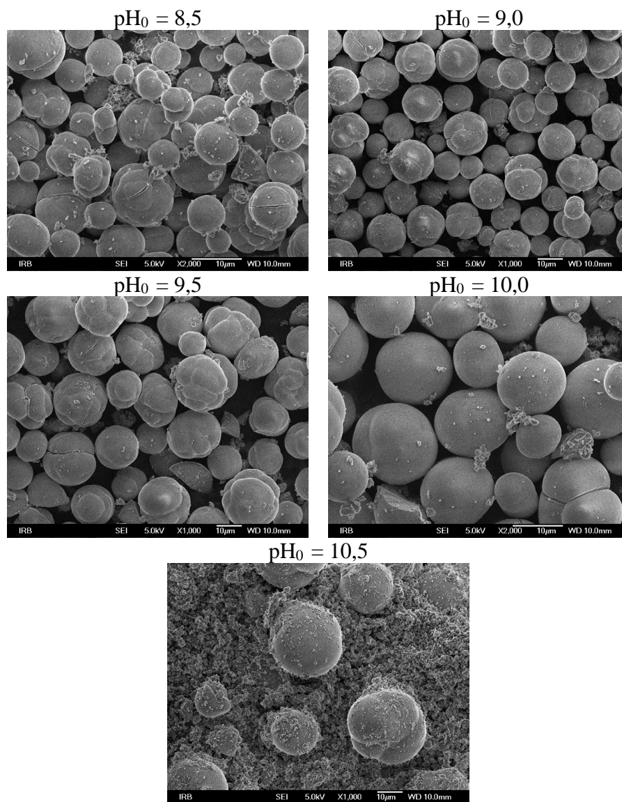
Slika 11. SEM snimke taloga iz pokusa spontanog taloženja kalcijeva karbonata pri različitim početnim pH vrijednostima u sustavima uz dodatak c(pAsp) = 5 ppm.
