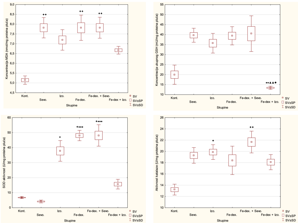
Slika 17. Koncentracija malondialdehida, ukupnog glutationa i aktivnost SOD i CAT u tkivu pluća štakora obrađenih inhalacijskim anestheticima i željezo dekstranom te njihovom kombinacijom
