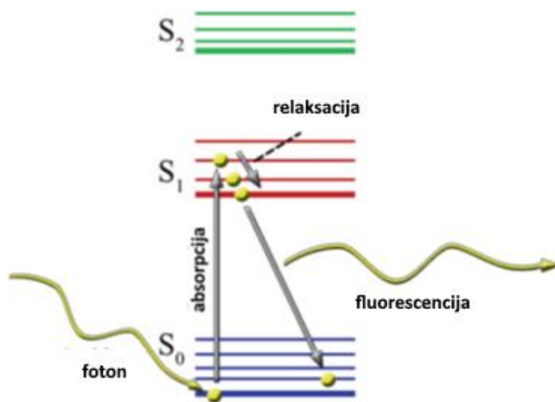
Slika 2. Jablonski dijagram elektronskog stanja pobuđene molekule i nastanka fluorescencije (preuzeto i prilagođeno iz izvora 24)
