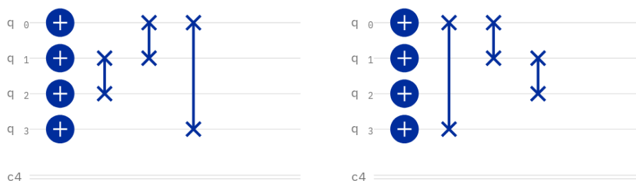
Slika 5.5: Kvantni krug koji mapira |x\rangle u |7^x \bmod 15\rangle (lijevo) odnosno u |13^x \bmod 15\rangle (desno). Slike su preuzete direktno iz IBM Quantum Composer -a.
