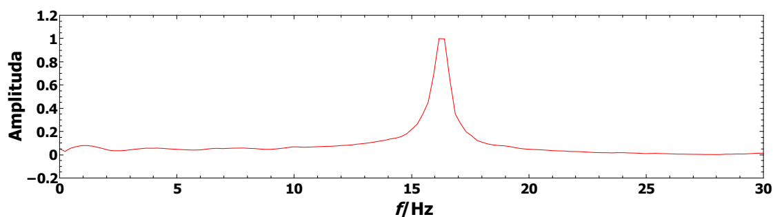
Slika 5.52: Prikaz frekvencijske karakteristike za titranje cilindra u postavu u kojem je Ugljikov dioksid volumena 65 ml. Vrh je na frekvenciji od 16,17 \pm 0,03 Hz.
