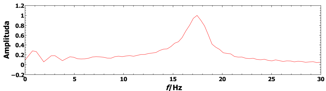
Slika 5.30: Prikaz frekvencijske karakteristike za titranje cilindra u postavu u kojem je Helij volumena 65 ml. Vrh je na frekvenciji od 17,43 \pm 0,03 Hz.
