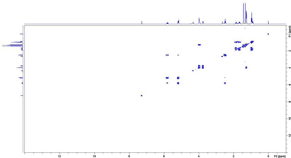
Slika D11. COSY NMR spektar spoja 8 u \text{CDCl}_3 .
