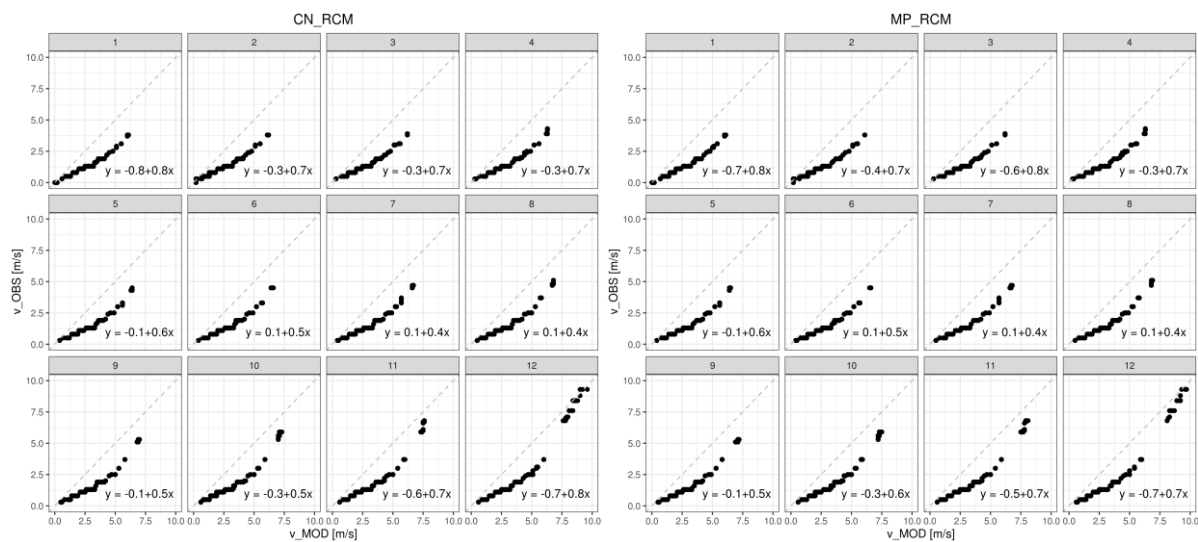
Slika S11c Odnos sortiranih vrijednosti brzine vjetra iz regionalnog modela REG forsiranog globalnim modelom CN (lijevo) i MP (desno) u odnosu na izmjerene vrijednosti s postaje Zagreb-Maksimir u razdoblju 1981. – 2010.
