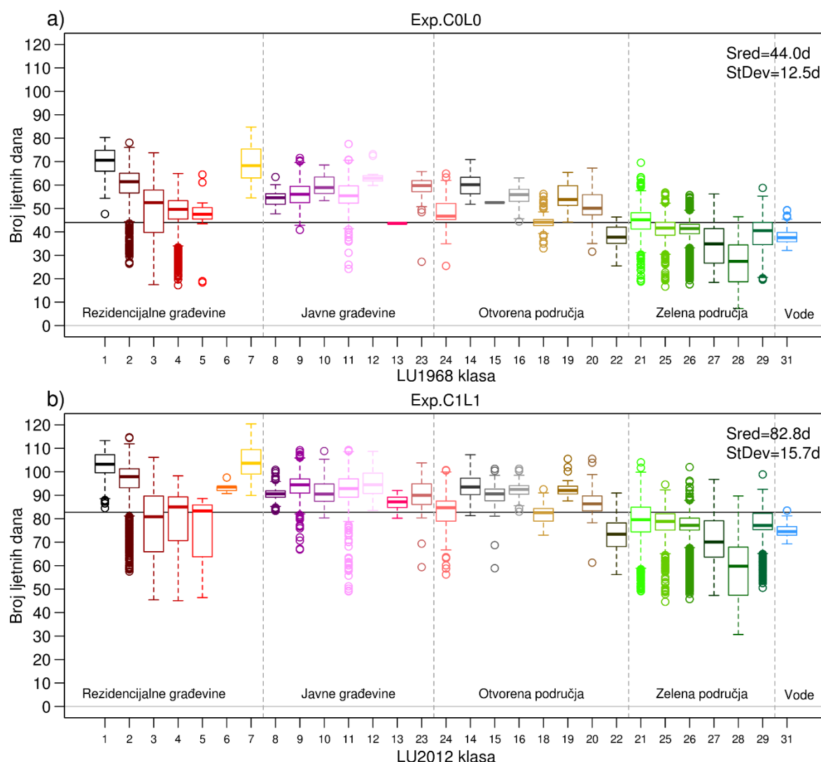
Slika 5.4.3 Prosječan broj ljetnih dana (Tx25) u uvjetima a) ranije situacije namjene zemljišta grada i ranijih klimatskih uvjeta (Exp.C0L0) i b) novije situacije namjene zemljišta i recentnih klimatskih uvjeta (Exp.C1L1). Crna horizontalna linija odgovara prosječnoj vrijednosti broja dana Tx25 za svaki od eksperimenata.
