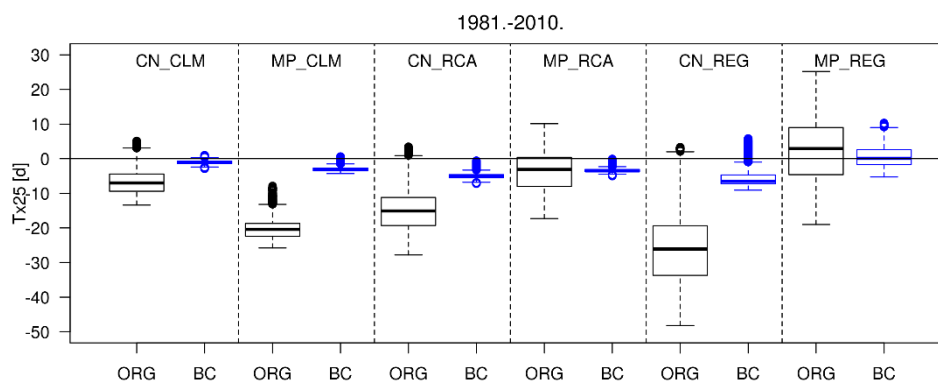
Slika 5.5.3 Razlika modeliranog prosječnog broja ljetnih dana (Tx25) na temelju izvornih podataka regionalnih modela (ORG) te nakon korekcije pristranosti (BC) u odnosu na kontrolno polje dobiveno na temelju podataka mjerenja s postaje Zagreb-Maksimir u razdoblju 1981. – 2010.
