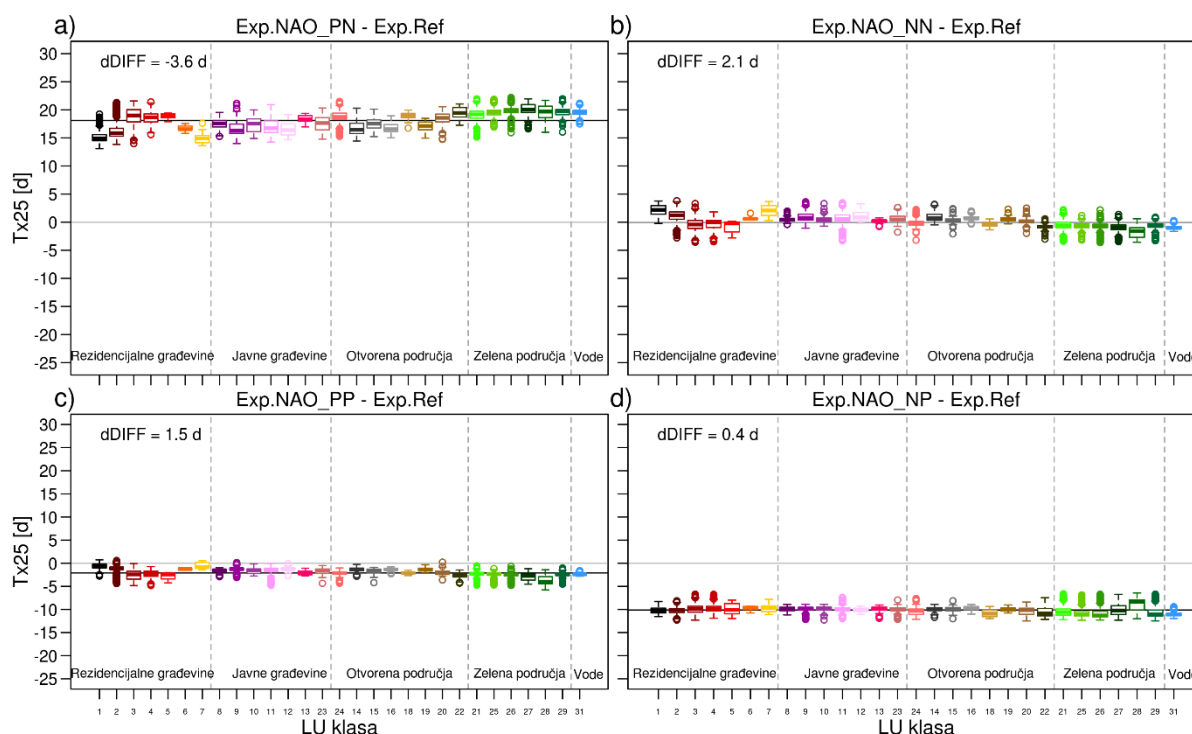
Slika 5.3.4 Promjena broja ljetnih dana (Tx25) u odnosu na referentnu situaciju (Exp.Ref) za:
