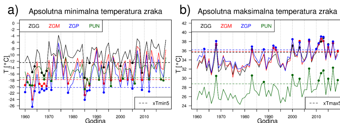
Slika 5.2.1 Godišnje apsolutne a) minimalne i b) maksimalne temperature zraka na postajama Zagreb-Grič (ZGG), Zagreb-Maksimir (ZGM), Zagreb-Pleso (ZGP) i Puntijarka (PUN) u razdoblju 1960. – 2019. Odgovarajuće 5-godišnje povratne vrijednosti označene su isprekidanom linijom, dok su premašaji tog praga označeni točkama.
