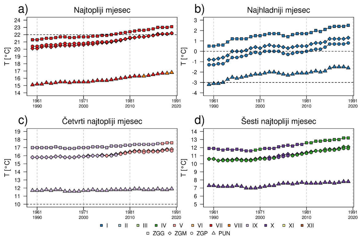
Slika 5.1.2 Prosječne vrijednosti temperature zraka a) najtoplijeg, b) najhladnijeg, c) četvrtog najtoplijeg i d) šestog najtoplijeg mjeseca za klizna 30-godišnja razdoblja u razdoblju 1960. – 2019. Odgovarajući kalendarski mjesec označen je bojom simbola, dok oblik simbola odgovara pojedinoj postaji.
