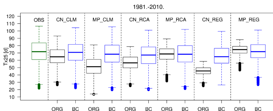
Slika 5.5.2 Modelirani prosječan broj ljetnih dana (Tx25) na području Zagreba u razdoblju 1981. – 2010. kada se kao ulazni podaci u kuboidnu metodu koriste mjerenja s postaje Zagreb-Maksimir (OBS), izvorni podaci regionalnih modela (ORG) te korigirani podaci regionalnih modela (BC).
