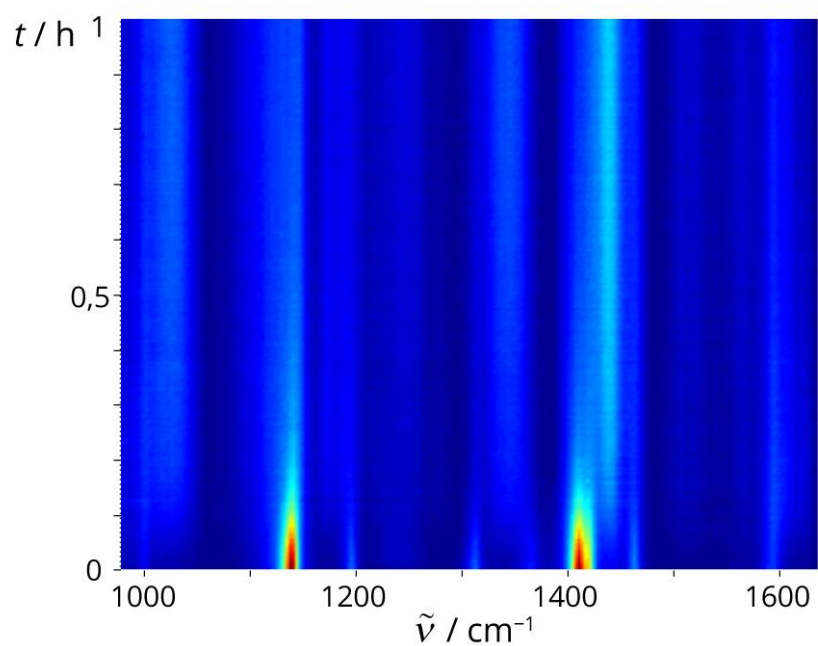
Slika D36. 2D prikaz vremenski razlučenog Ramanovog praćenja NG reakcije L7 (0,5 mmol) s NCS-om (0,6 mmol) i SiO 2 (250 mg).
