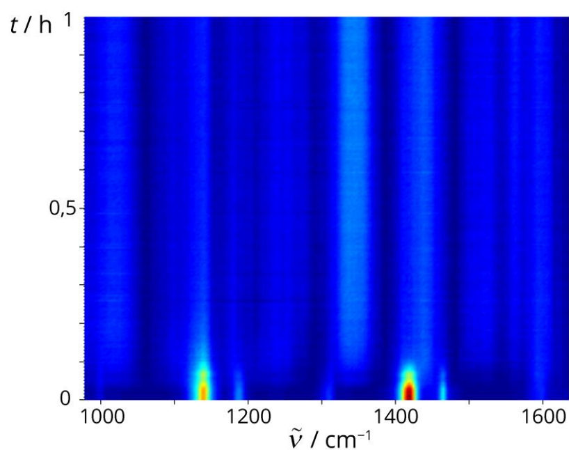
Slika D35. 2D prikaz vremenski razlučenog Ramanovog praćenja NG reakcije L6 (0,5 mmol) s NIS-om (0,6 mmol) i SiO 2 (250 mg).
