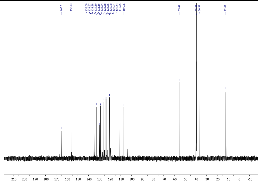
Slika D55. ^{13}\text{C} NMR spekter ( E )-3-etiliden-2-(2-metoksibenzil)izoindolinona ( E -2h)
