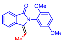
Slika 35. Strukturna formula molekule spoja E-2o
