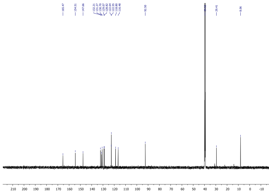
Slika D15. ^{13}\text{C} NMR spektar 3-etil-3-hidroksi-2-(2-hidroksifenil)izoindolinona (1k)
