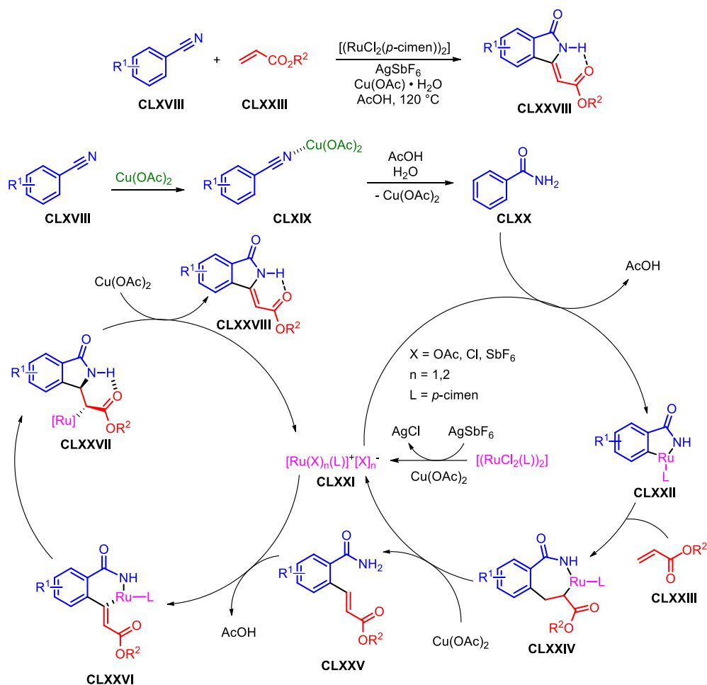
Shema 28. Priprava Z-3-metilenizindolinona katalizirana rutenijevim kompleksom [(\text{RuCl}_2(p\text{-cimen}))_2]
