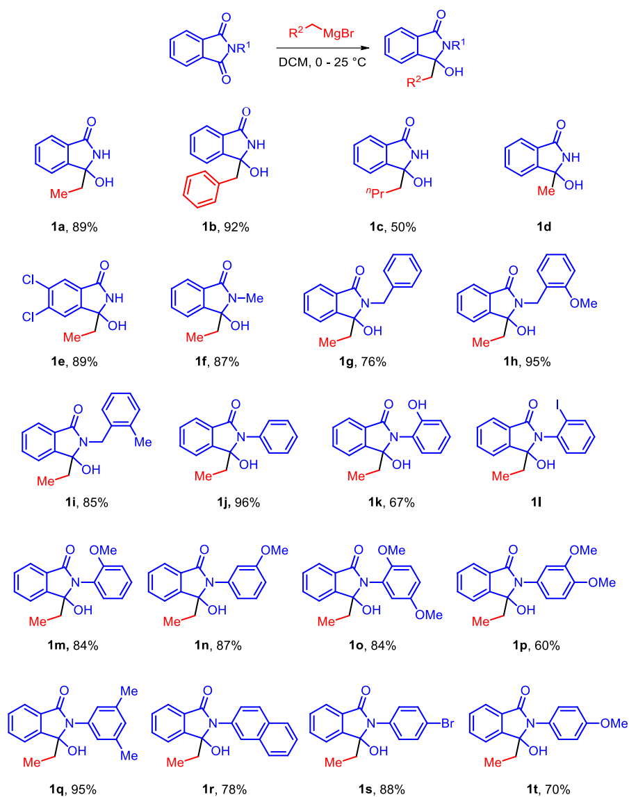
Slika 44. Priprava 3-alkil-3-hidroksiizoinolinona
