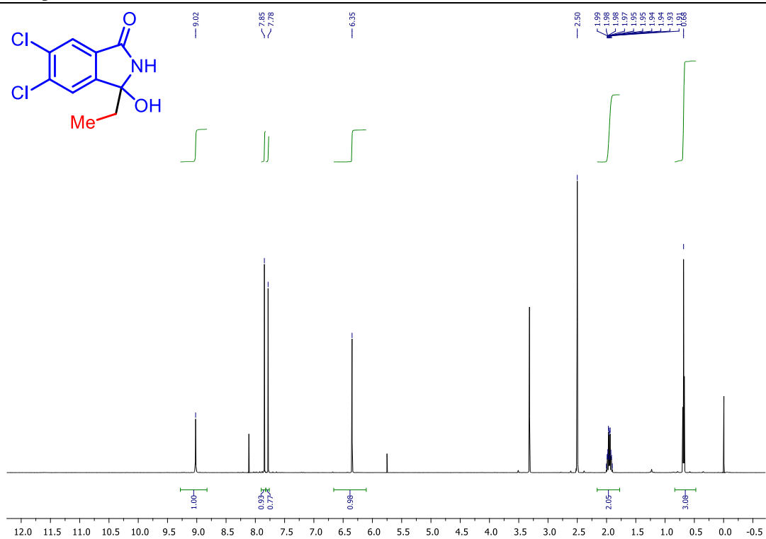
Slika D2. 1 H NMR spektar 5,6-diklor-3-etil-3-hidroksiizoinolinona ( 1e )
