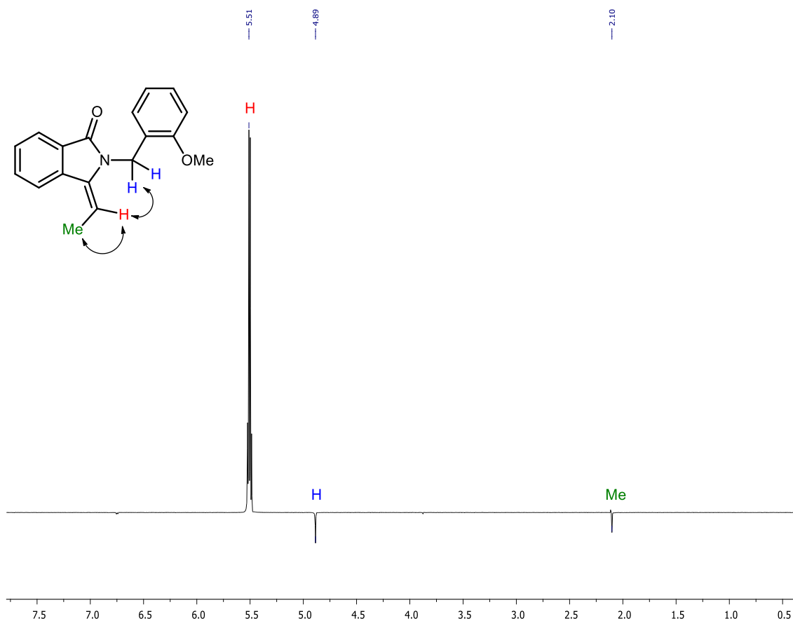
Slika D56. Selektivni NOESY spekter koji pokazuje H-H i H-H interakcije in E -2h
