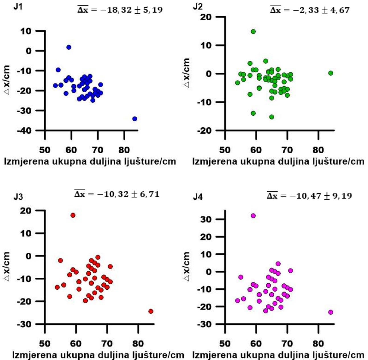
Slika 10. Grafički prikaz razlike između izmjerene i izračunate ukupne dužine školjke ( \Delta x ) za pojedinačne formule za izračun ukupne duljine ljušture iz nezakopanog dijela ljušture. Svaki dio slike grafički prikazuje jednu formulu: J1) De Gaulejac i Vicente, 1990; J2) Garcia March i Ferrer, 1995; J3) Garcia-March, 2006; J4) Tempesta i sur., 2013. U gornjem desnom kutu svakog grafa je prikazana srednja vrijednost i standardna devijacija za pojedinačnu jednadžbu.
