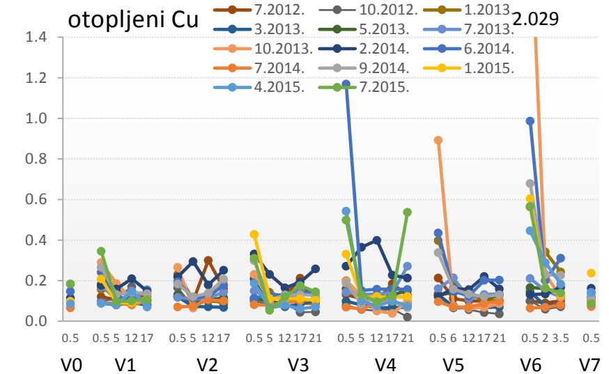
Slika 24. Ukupne i otopljene koncentracije Cs i Cu u vodi Visovačkoga jezera. Na x-osi prikazane su lokacije i dubine uzoraka vode (0,5; 5; 12; 17 i 21 m).
