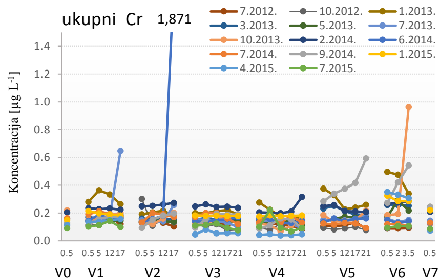
Slika 23. Ukupne i otopljene koncentracije Co i Cr u vodi Visovačkoga jezera. Na x-osi prikazane su lokacije i dubine uzoraka vode (0,5; 5; 12; 17 i 21 m).
