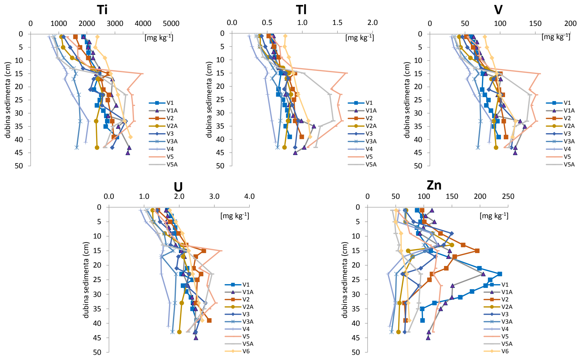
Slika 12. Raspodjela Ti, Tl, V, U i Zn u sedimentima Visovačkog jezera.
