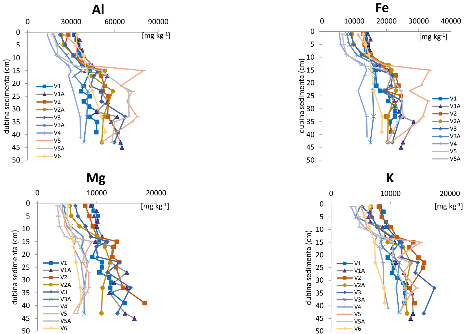
Slika 7. Raspodjela Al, Fe, Mg i K u sedimentima Visovačkoga jezera.
