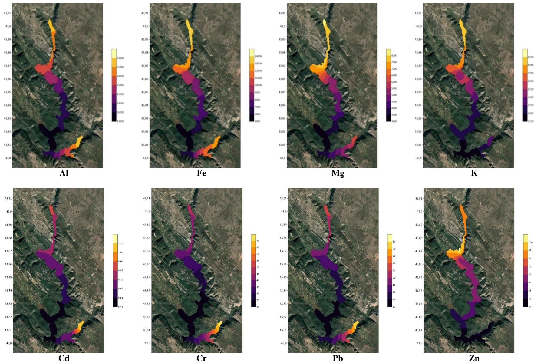
Slika 13. Prostorne raspodjele koncentracije [mg kg -1 ] glavnih i antropogenih elemenata u površinskim slojevima sedimenata.
