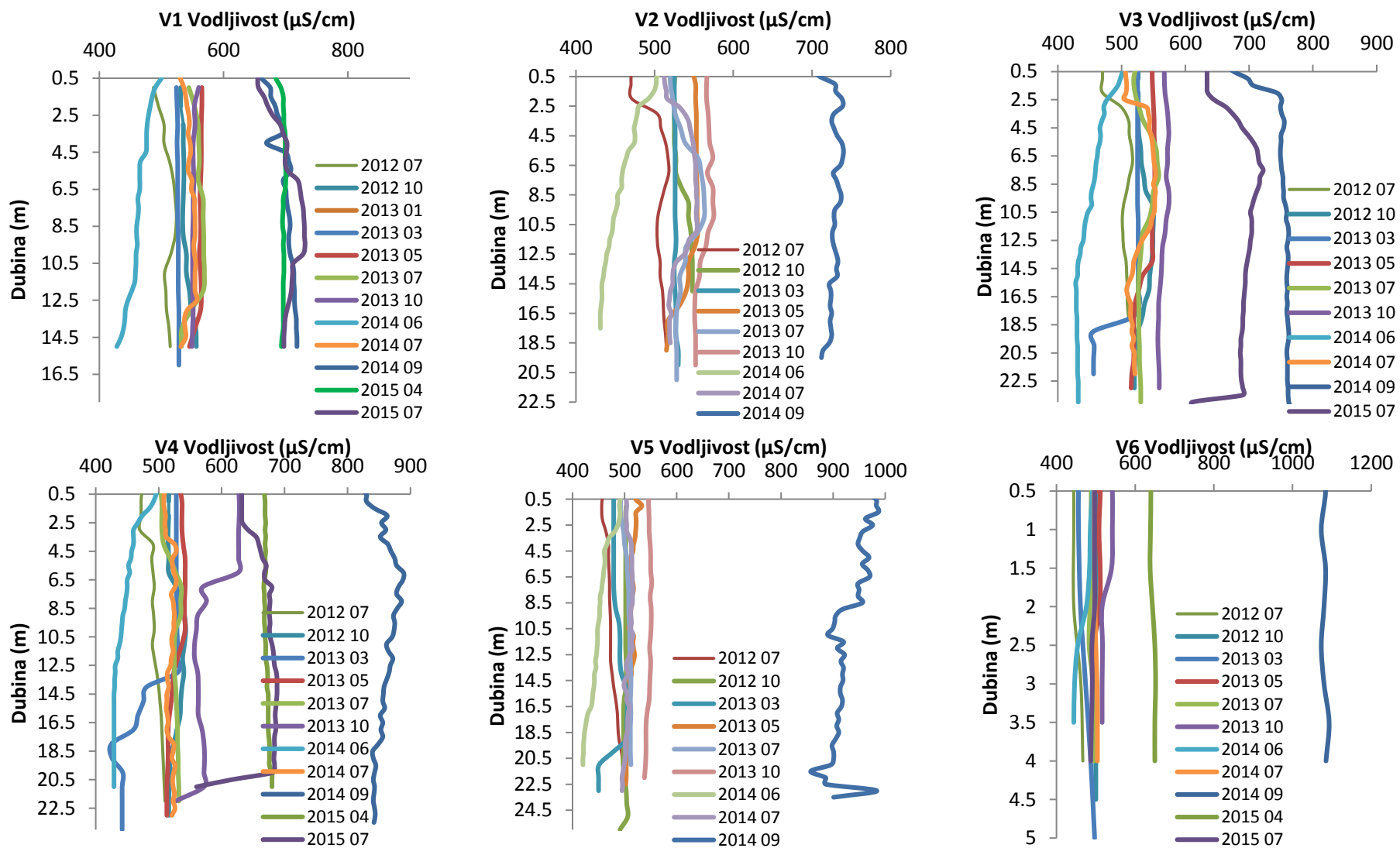
Slika 18. Vertikalni profili vodljivosti u vodi Visovačkoga jezera.
