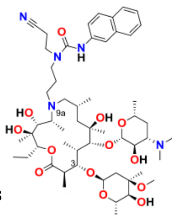
Slika 35. Strukturne formule molekula spojeva 47 i 48 i određene vrijednosti IC_{50} (a - osjetljivi soj, b - soj rezistentan na klorokin). 1
