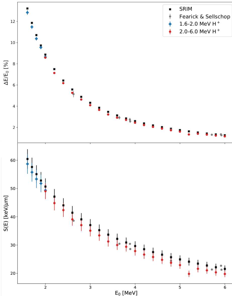
Slika 4.4: Graf ovisnosti gubitka energije u dijamantu u ovisnosti o početnoj energiji protonskog snopa ( gore ) i graf ovisnosti zaustavne moći u dijamantu o početnoj energiji protonskog snopa ( dolje ).
