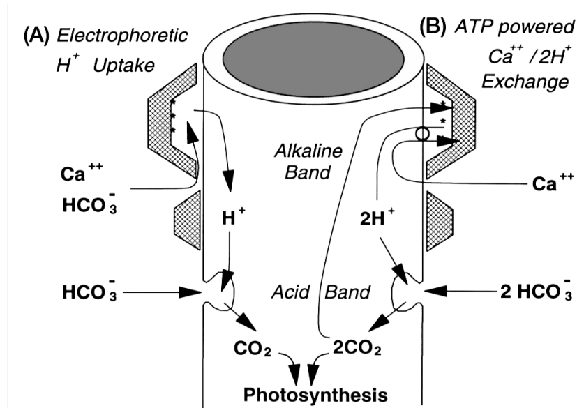
Slika 2. Shematski prikaz kalcifikacijskog modela alge roda Chara . (A) protonska elektroforeza pokrenuta membranskim električnim potencijalom. (B) Ca^{2+} - 2H^+ protutransport kataliziran Ca^{2+} -ATPazom. Preuzeto iz McConnaughey 1998.
